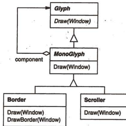
图2-7 MonoGlyph类关系
