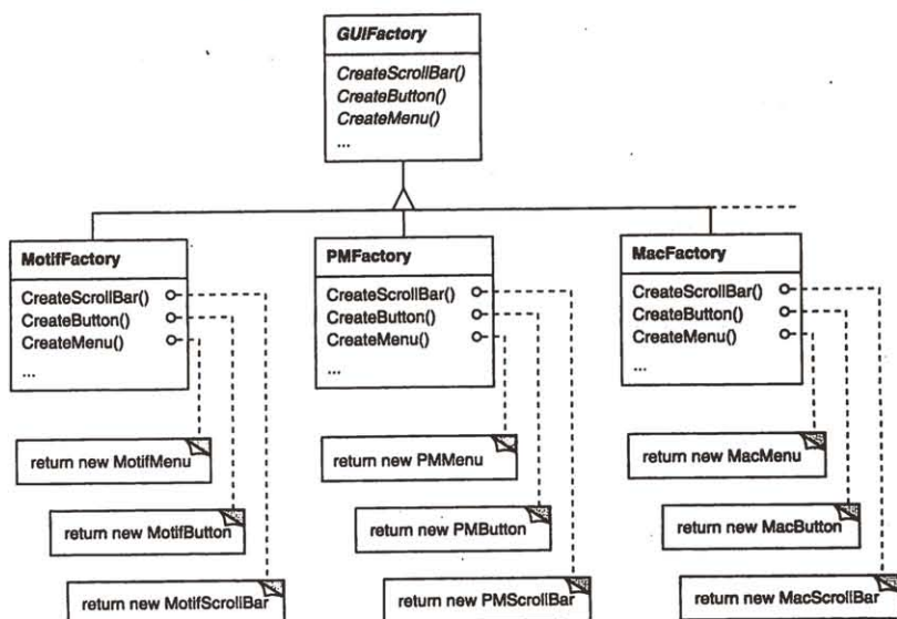
图2-9 GUIFactory类层次
