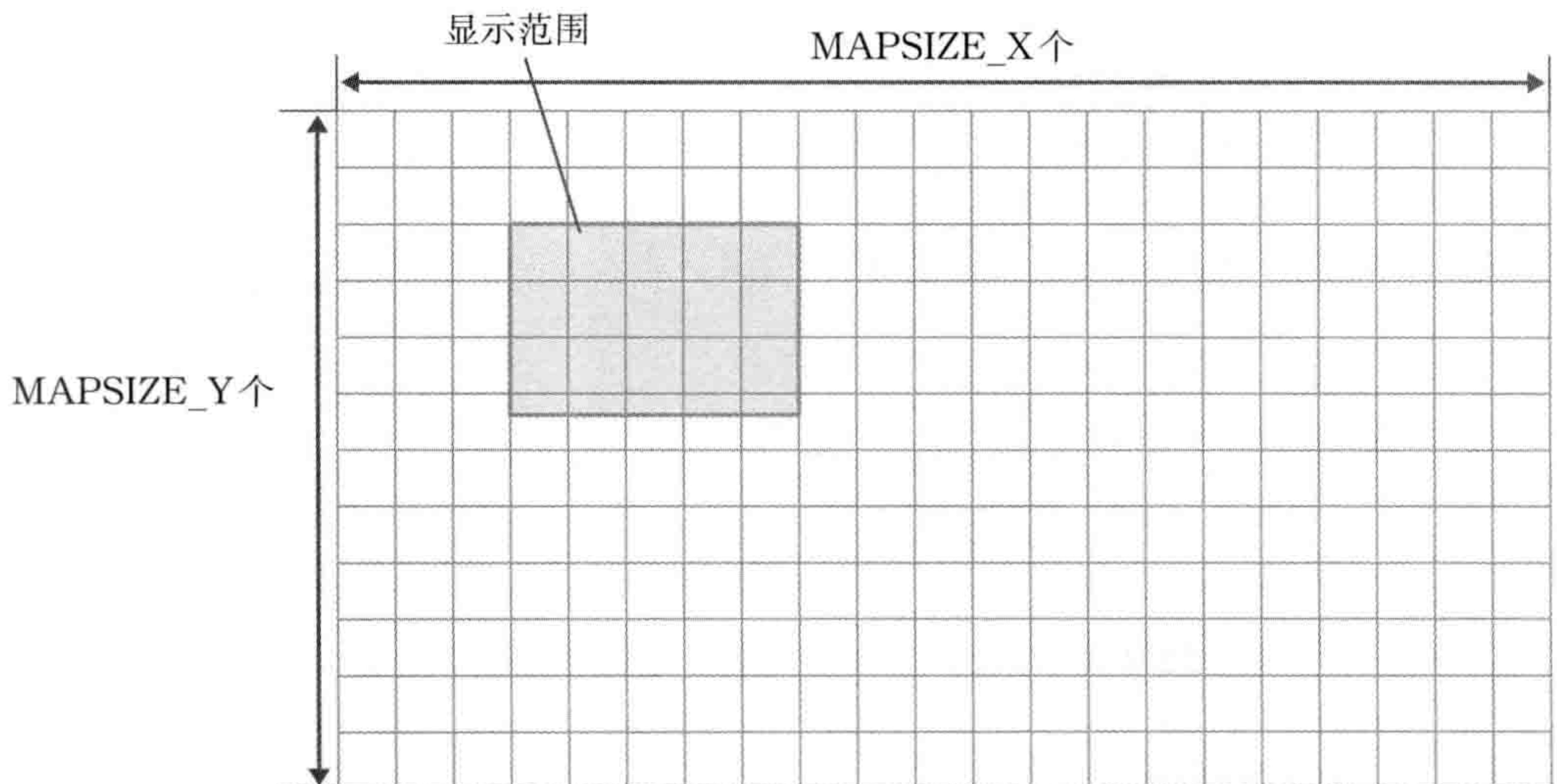
图2-3-2 从左上角坐标开始循环配置地图块
