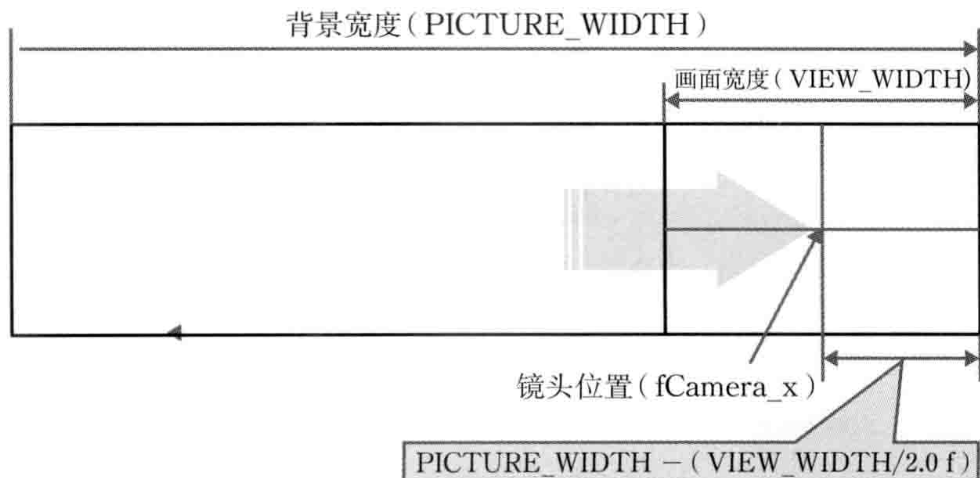
图2-1-3 画面到达背景的右端
