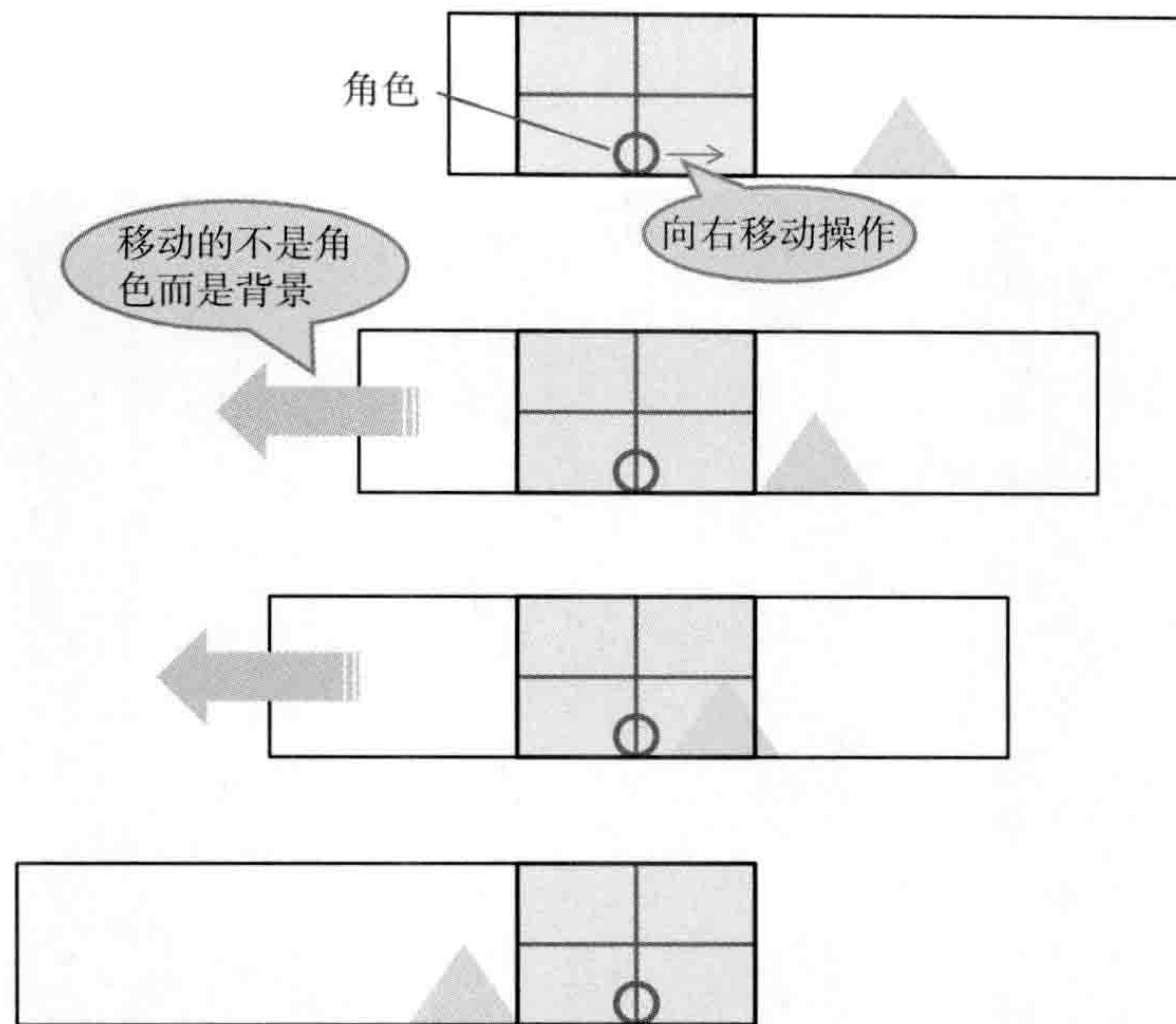
图2-2-2 根据角色操作只移动背景
