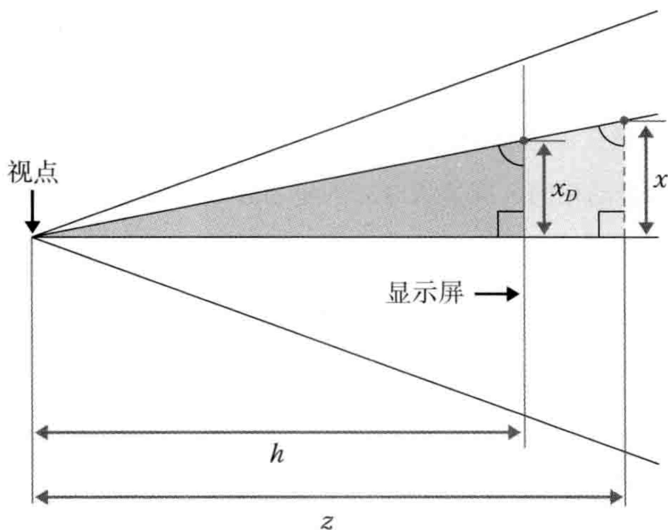
图2-6-1 3D中使用的视景物
