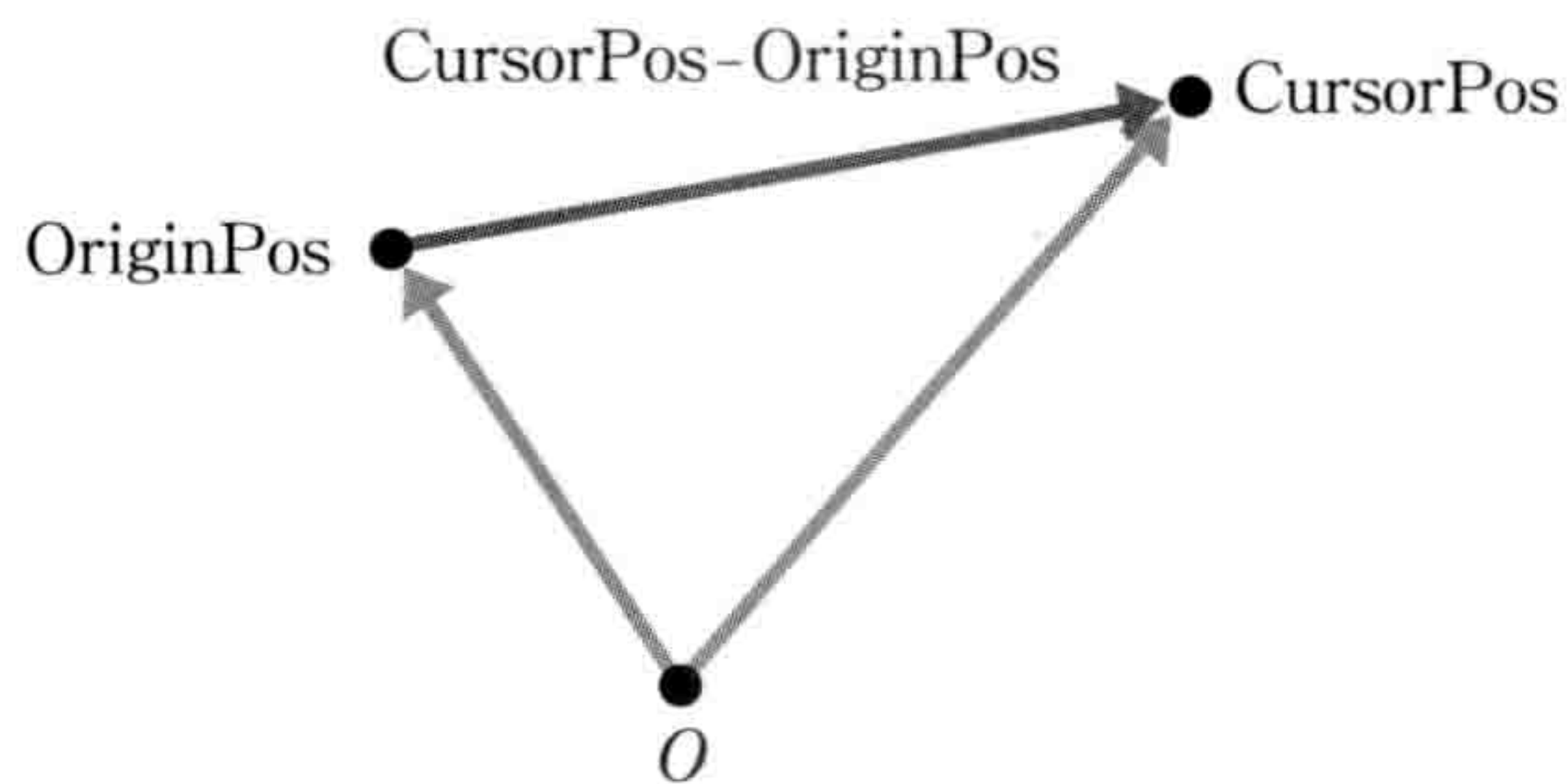
图 4-1-6 通过坐标间的减法得到坐标间的向量
