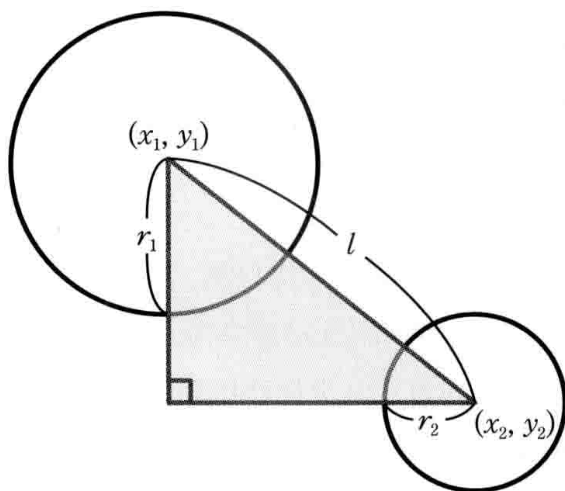
图3-2-3 根据勾股定理计算两圆圆心距离
