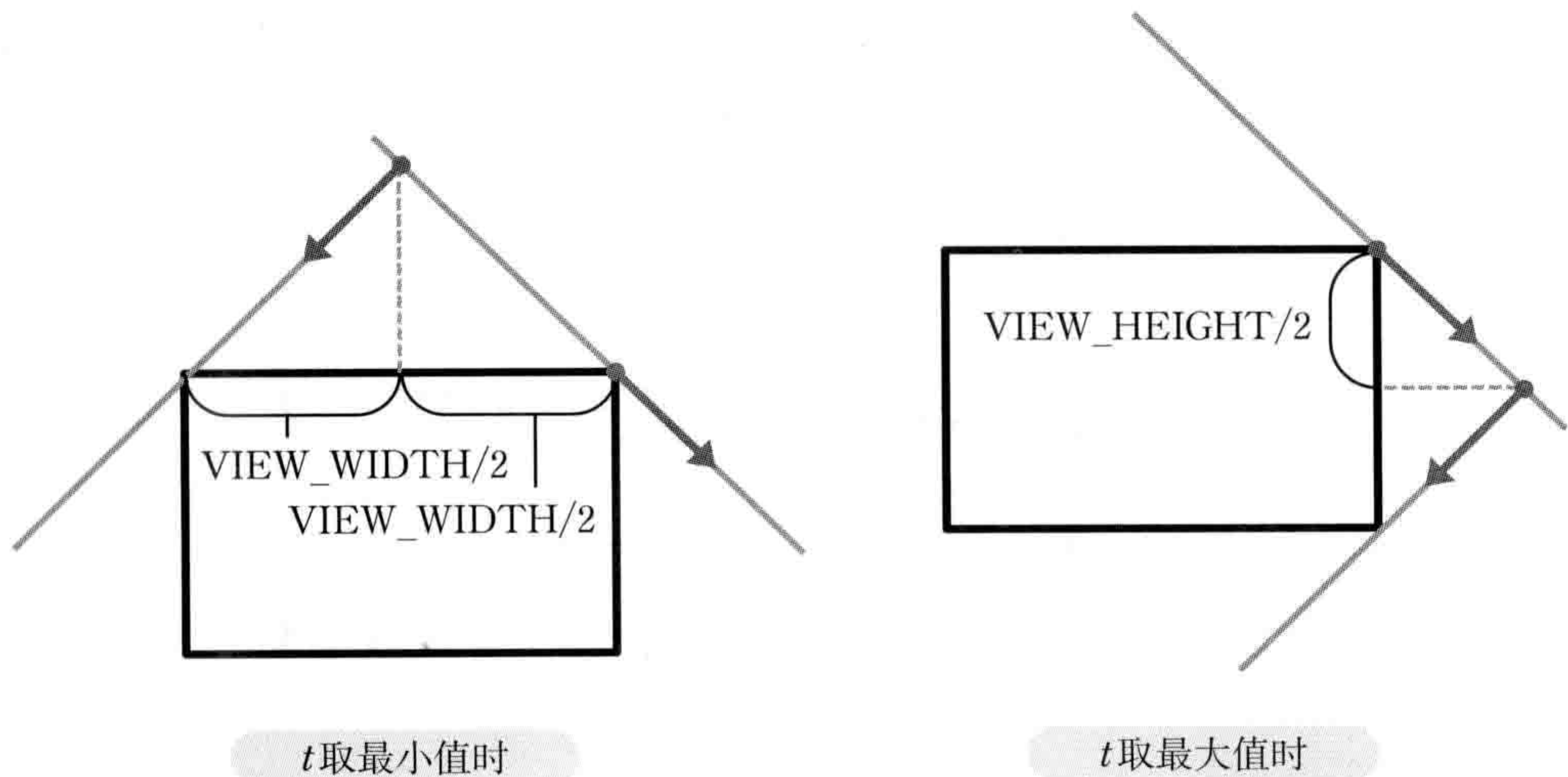
图5-2-3 t 的最大值与最小值
