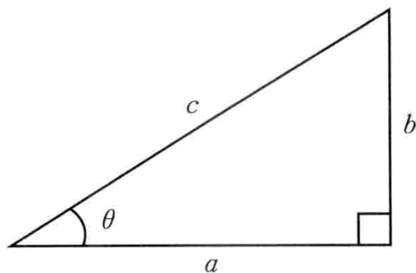
图6-4-1 直角三角形的三边与角 \theta
