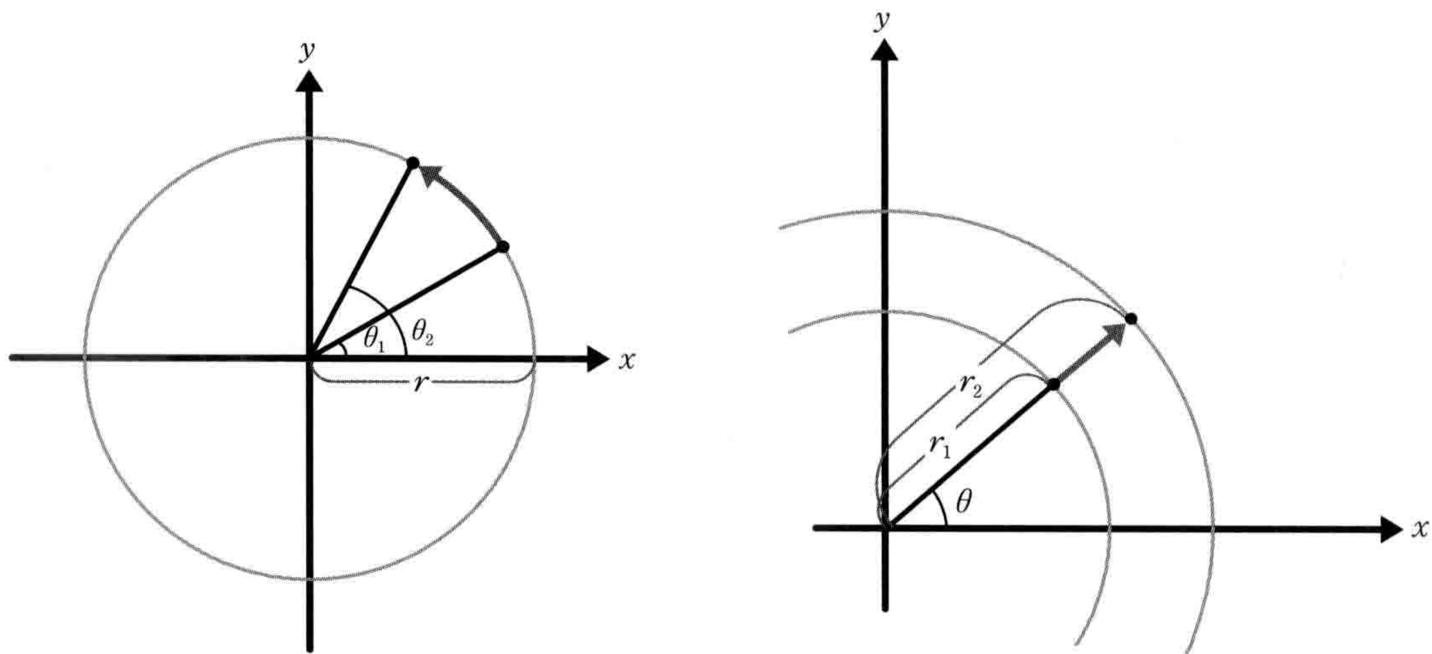
图6-4-3 使用三角函数移动坐标
