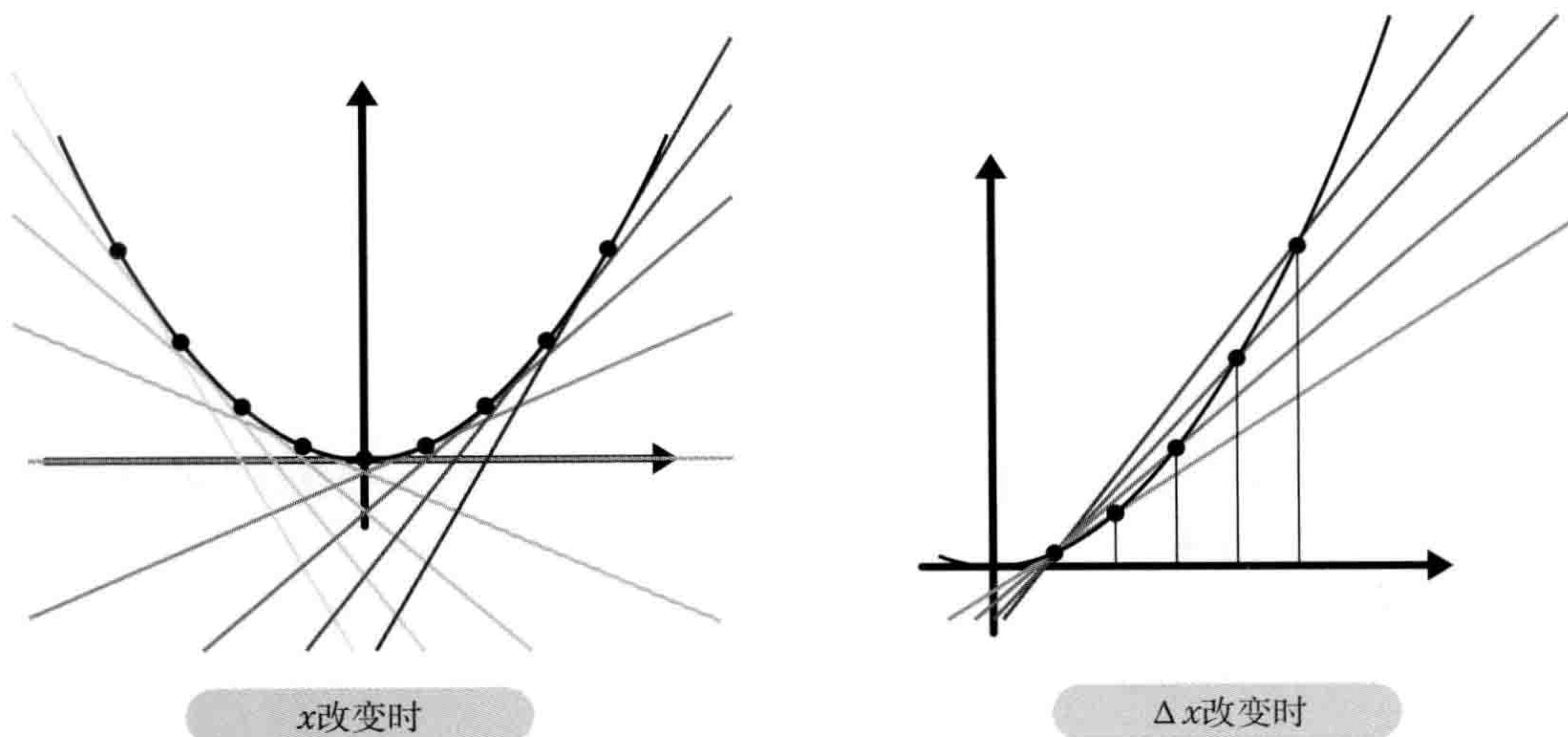
图6-6-1 抛物线 f(x) = ax^2 的变化率
