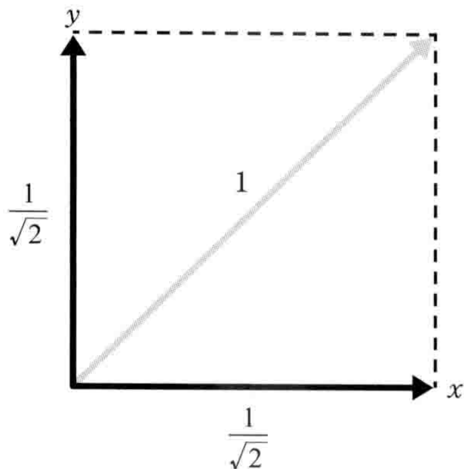
图1-2-5 重置物体在水平及垂直方向的移动速度为 \frac{1}{\sqrt{2}} ，使物体在斜方向上的移动速度保持不变
