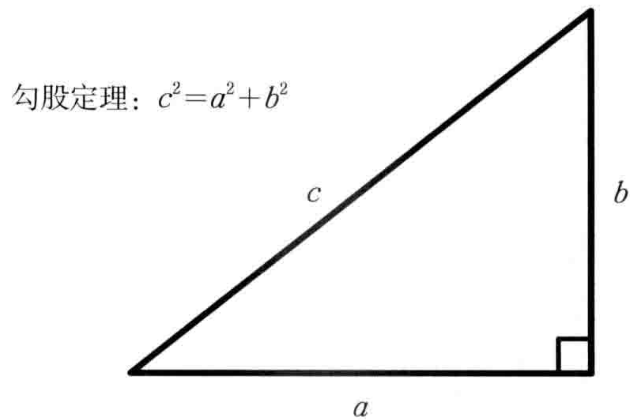
图1-2-3 通过两边的长度求剩余一边的长度
