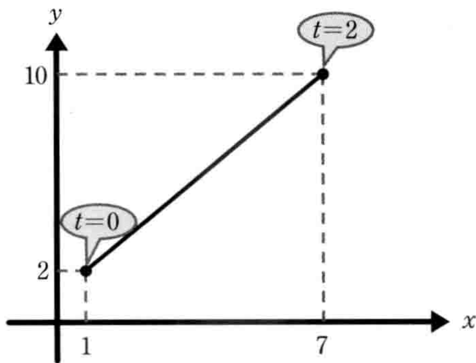
图6-1-4 连接点 (1, 2) 到点 (7, 10) 的线段
