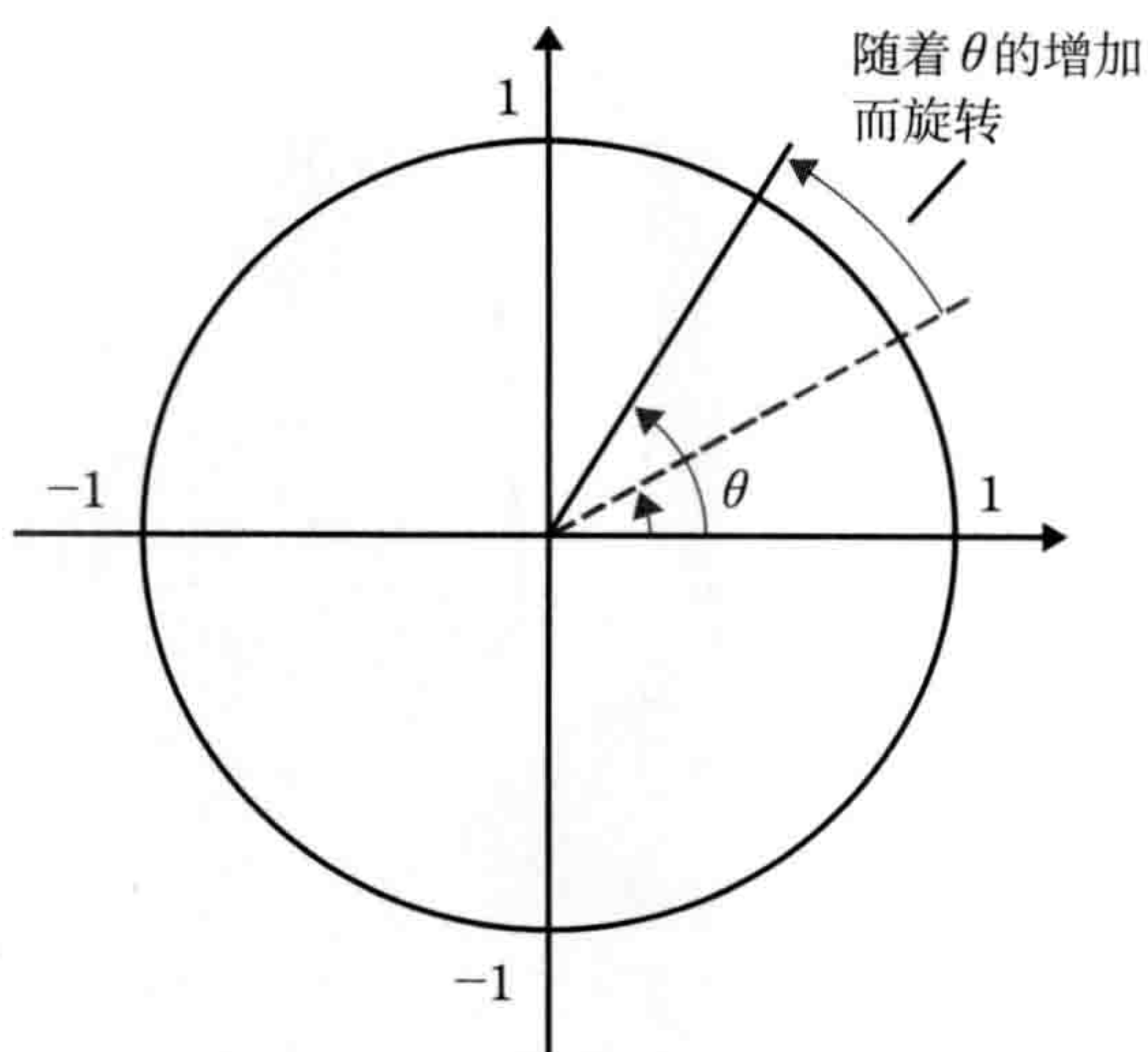
图 1-6-3 伴随时间进行的圆周运动
