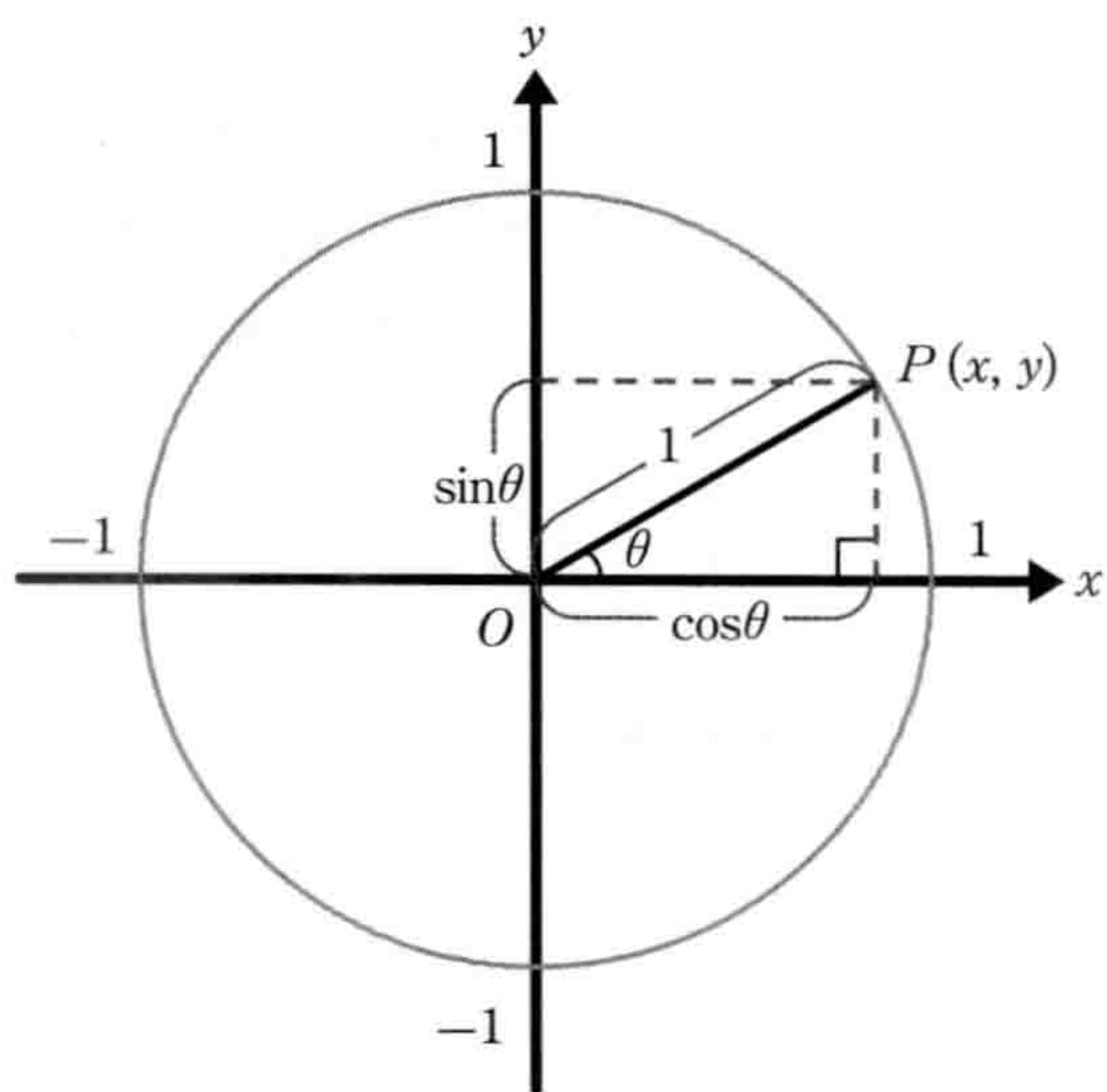
图6-4-4 基于单位圆的三角函数
