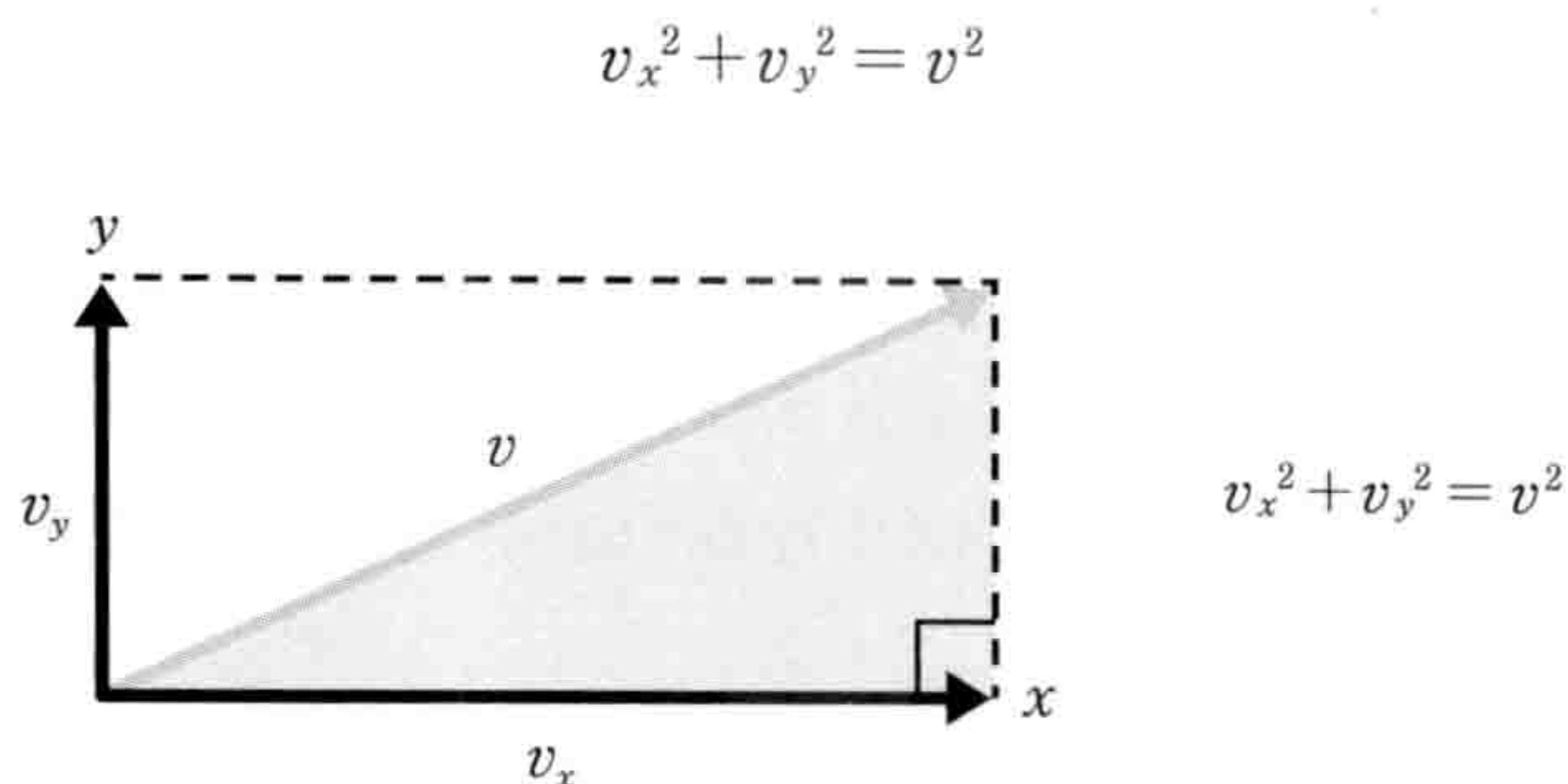
图1-3-3 对速度套用勾股定理
