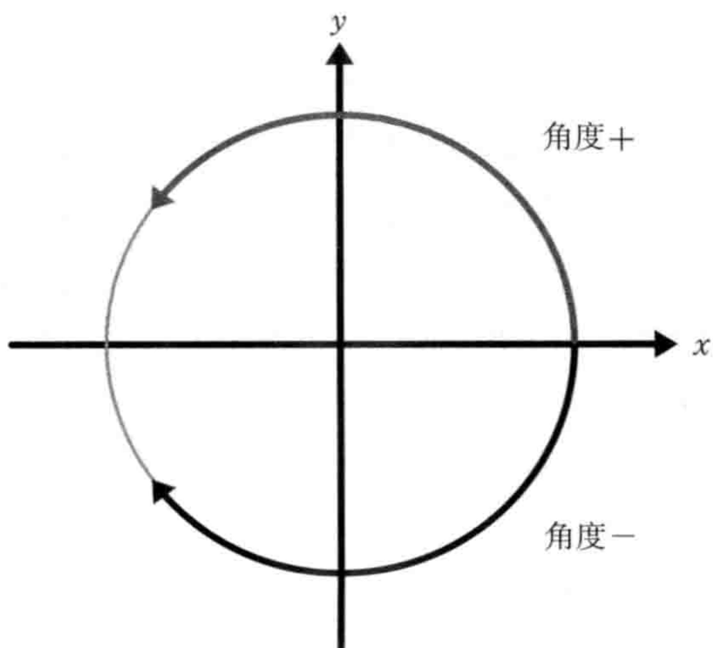
图6-4-6 负角
