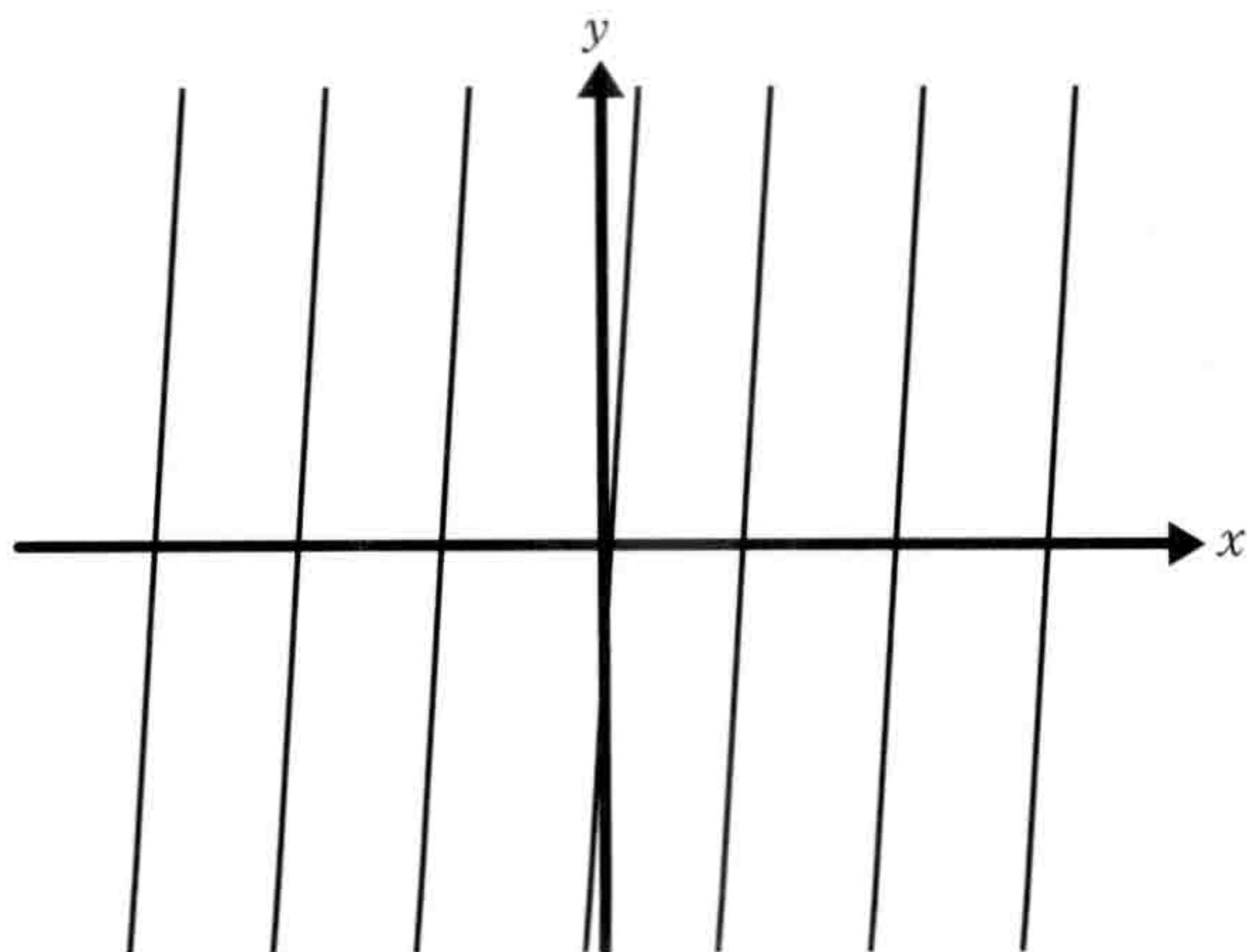
图6-1-3 相对于 y 轴有微小倾斜的直线
