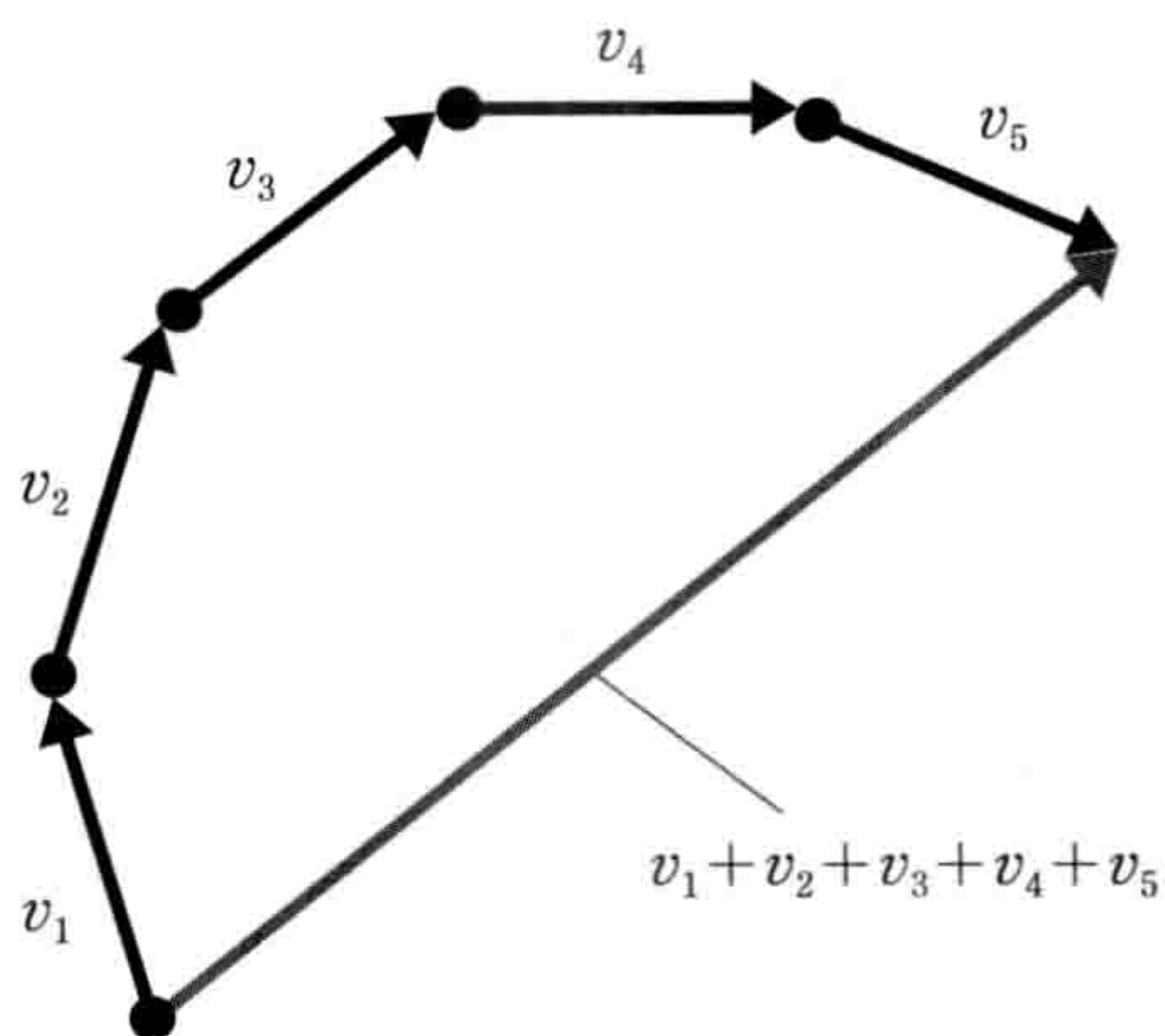
图6-5-1 向量的加法运算
