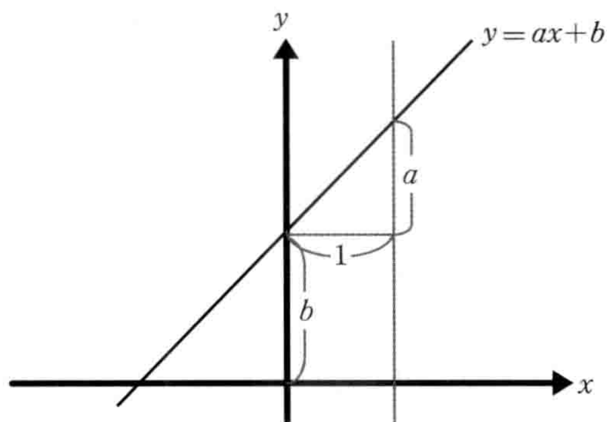
图6-1-2 一次函数的图形
