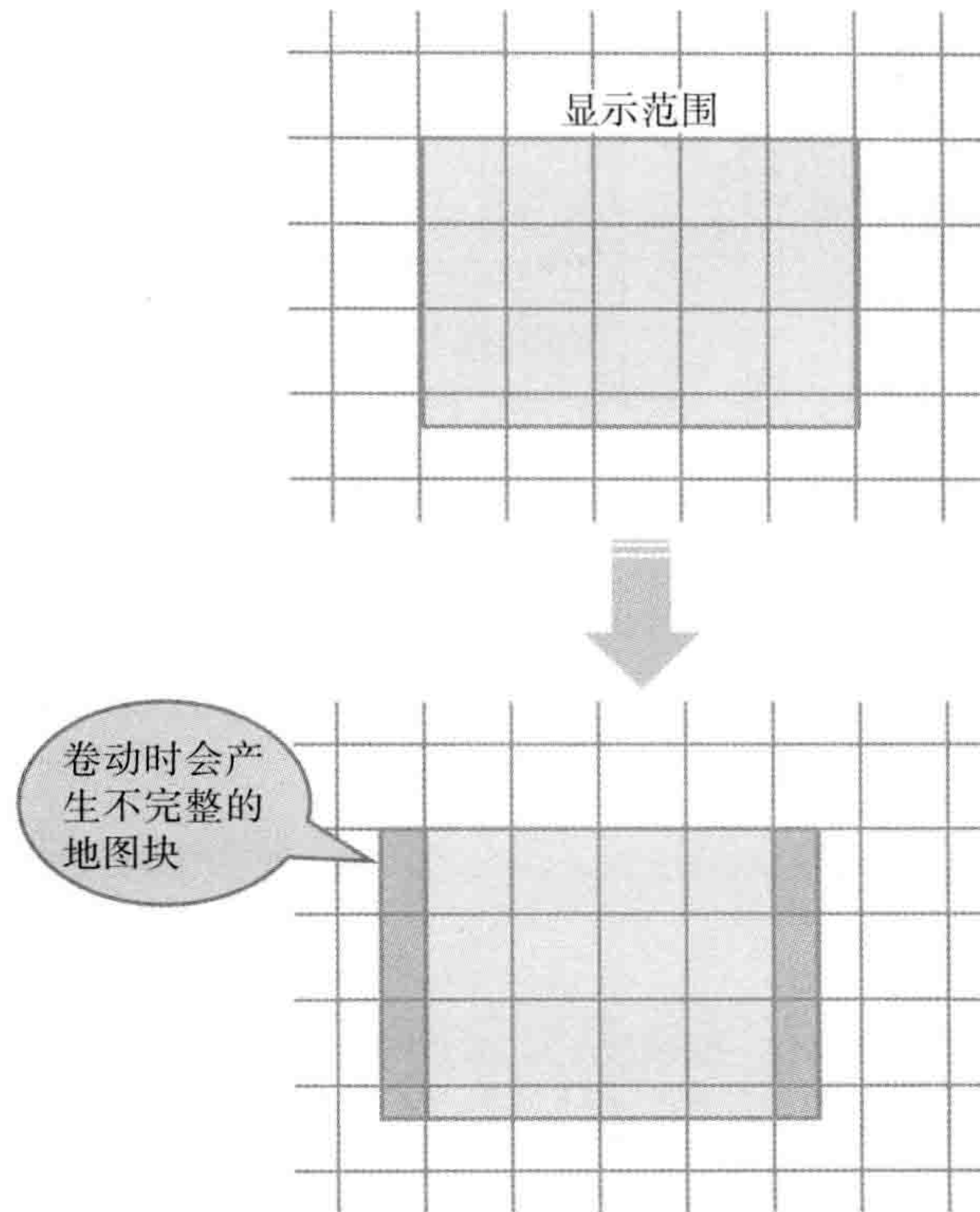
图2-3-6 滚动时会出现不完整的地图块
