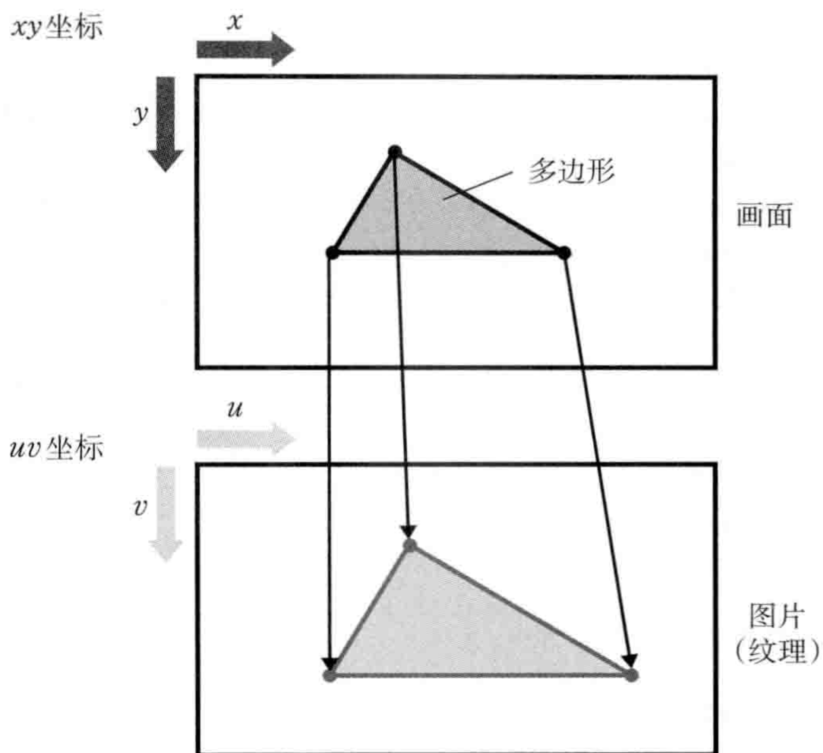
图5-1-2 通过 uv 坐标实现多边形的顶点与图片中的坐标相对应
