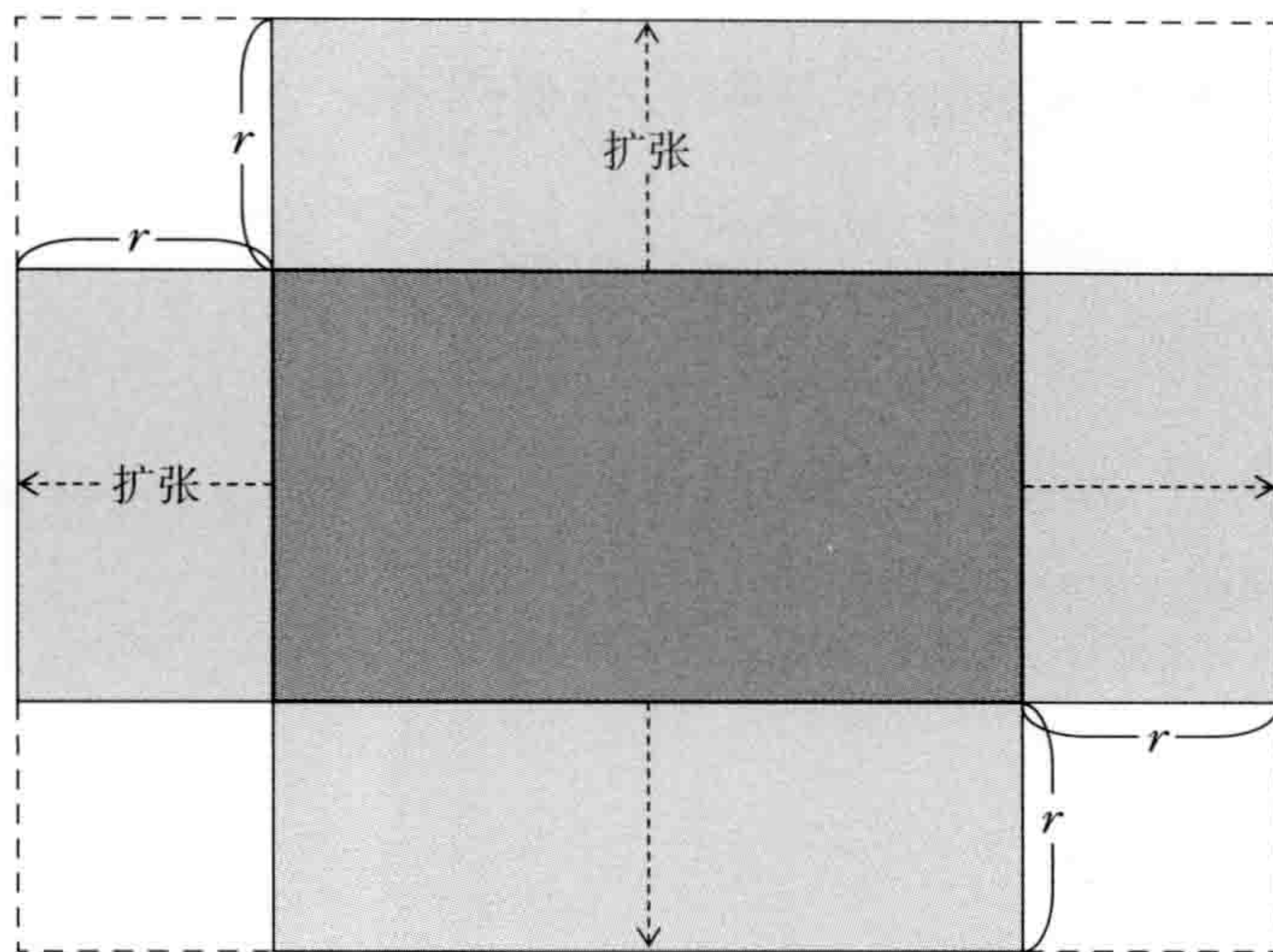
图3-2-4 将长方形向外扩张圆半径 r 来进行碰撞检测
