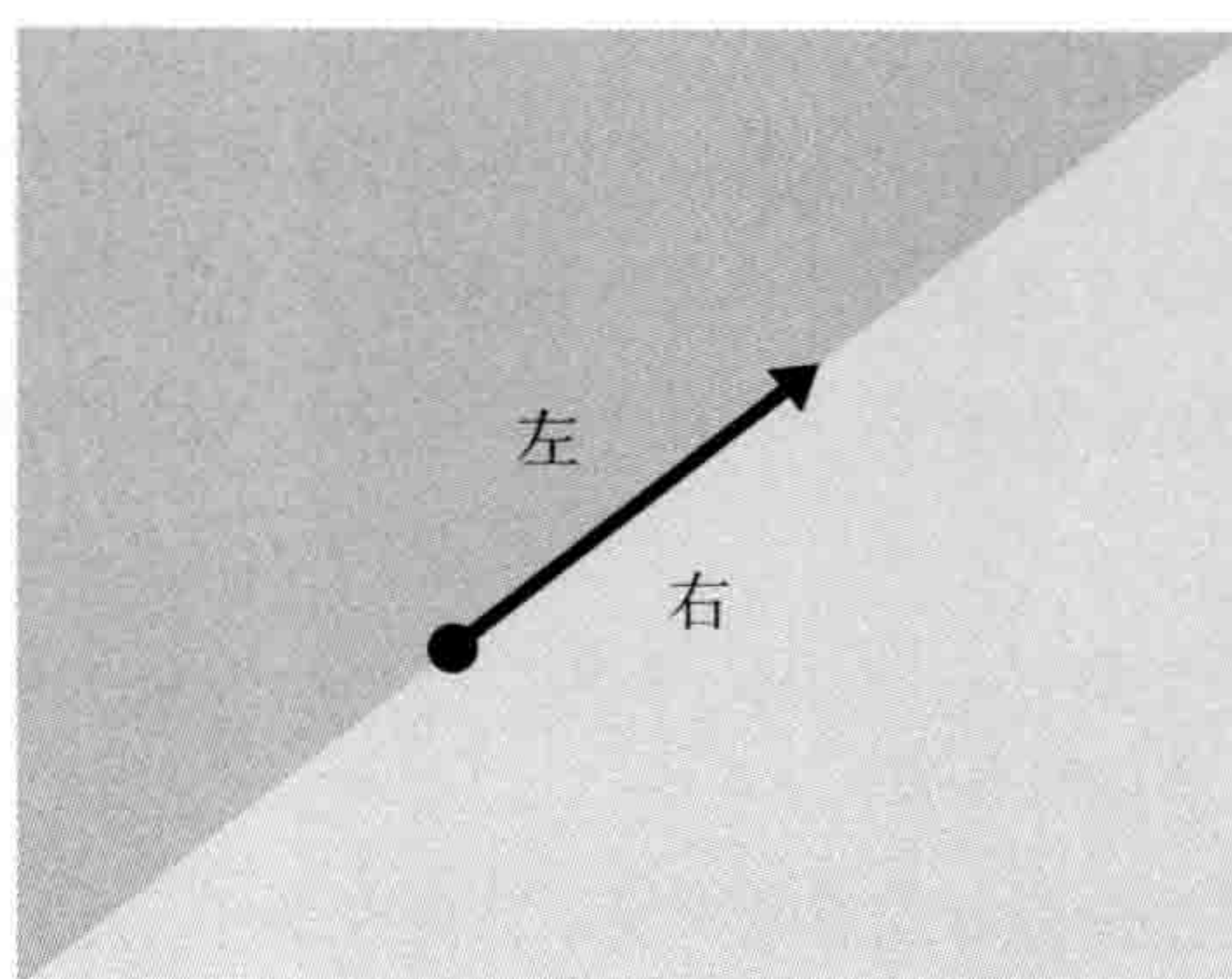
图4-4-3 一个点在线段的左侧还是右侧
