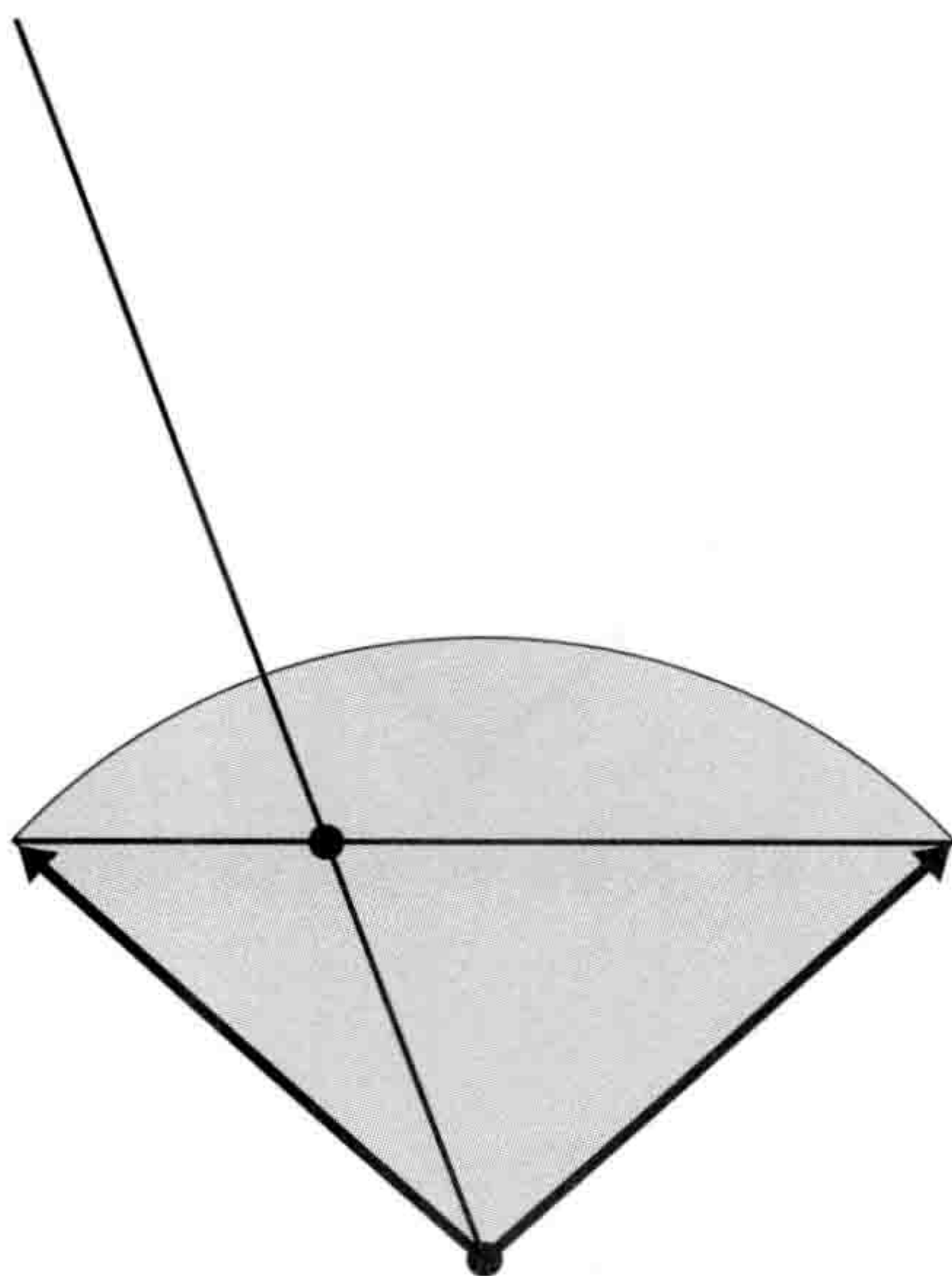
图3-4-5 通过内分点的射线
