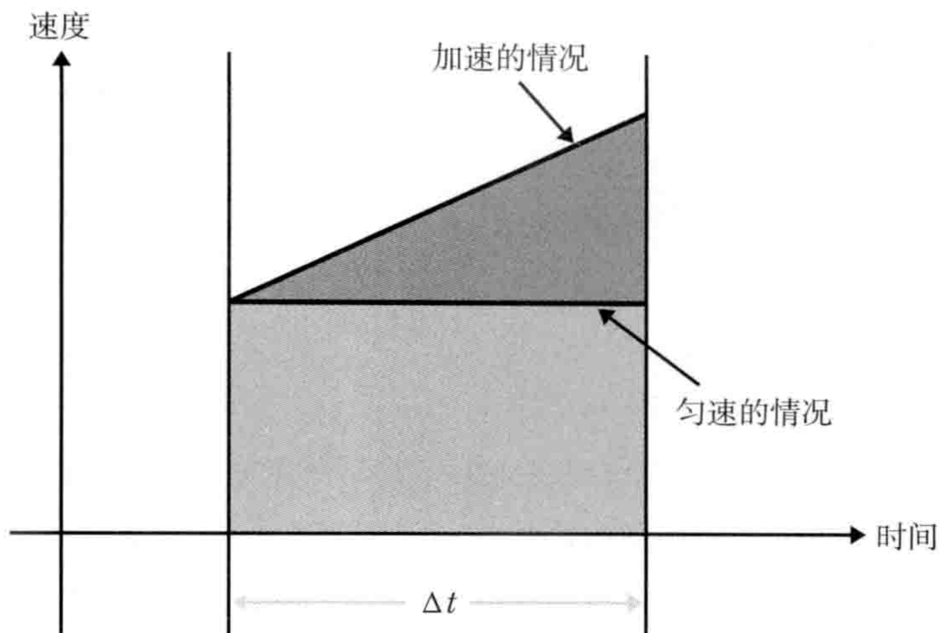
图1-4-2 匀速与加速时经过相同时间后产生的差异
