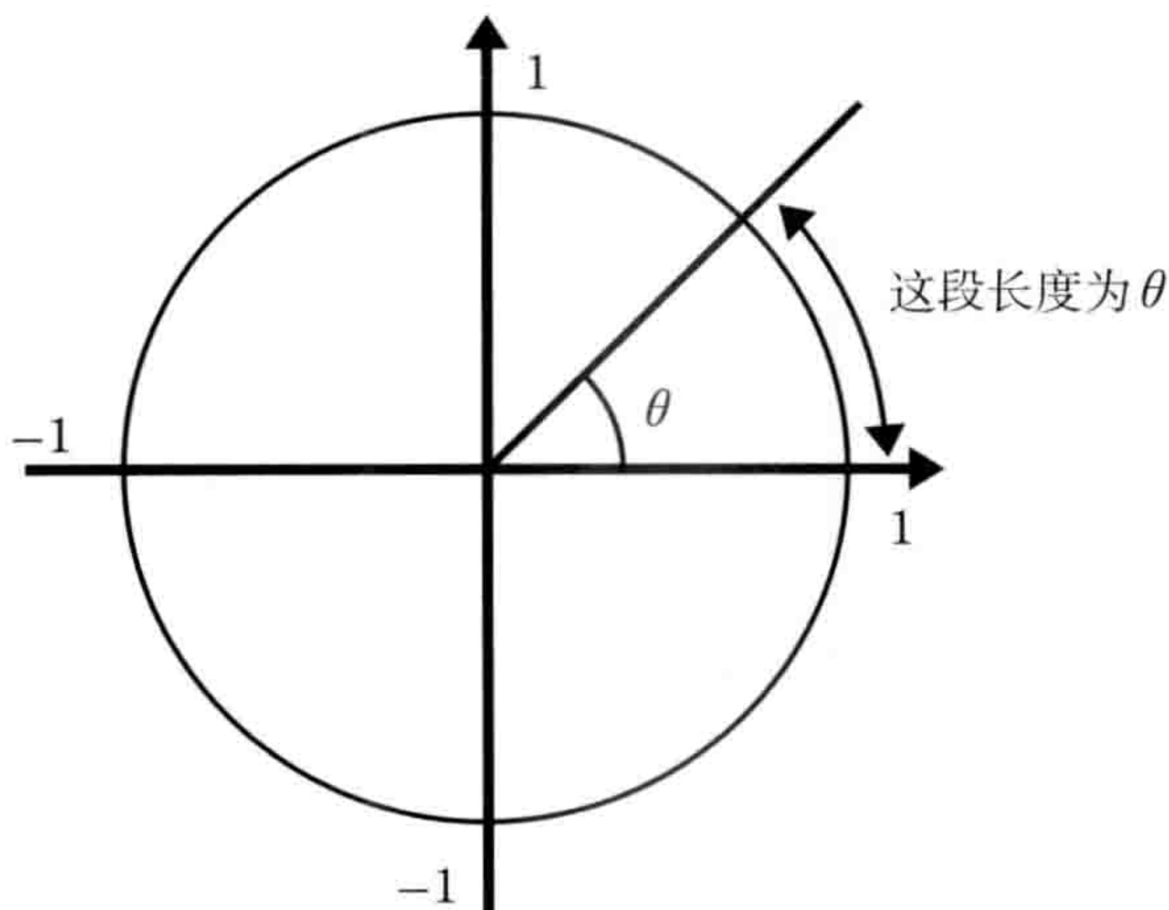
图1-3-5 弧度
