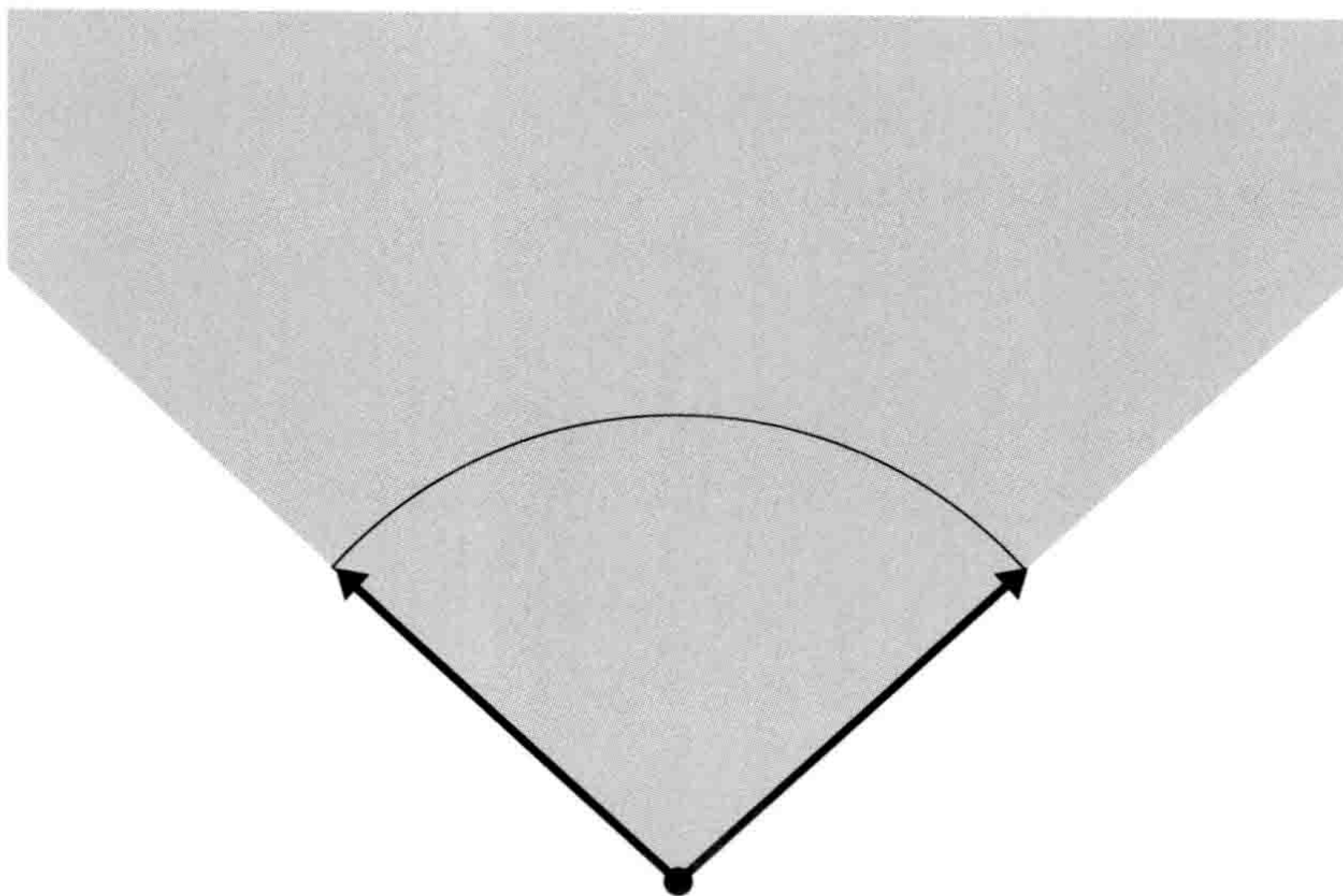
图3-4-6 向量 a 与向量 b 之间的范围
