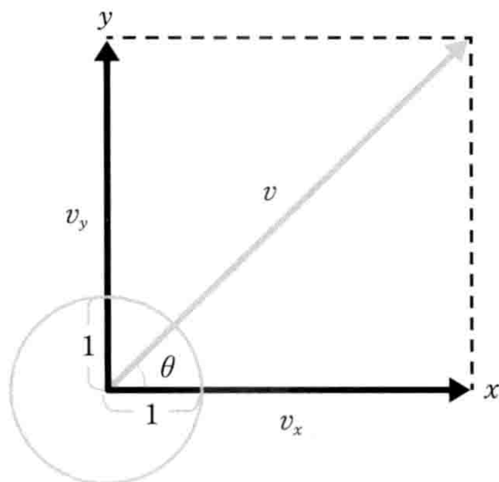
图1-3-4 单位圆与角度 \theta
