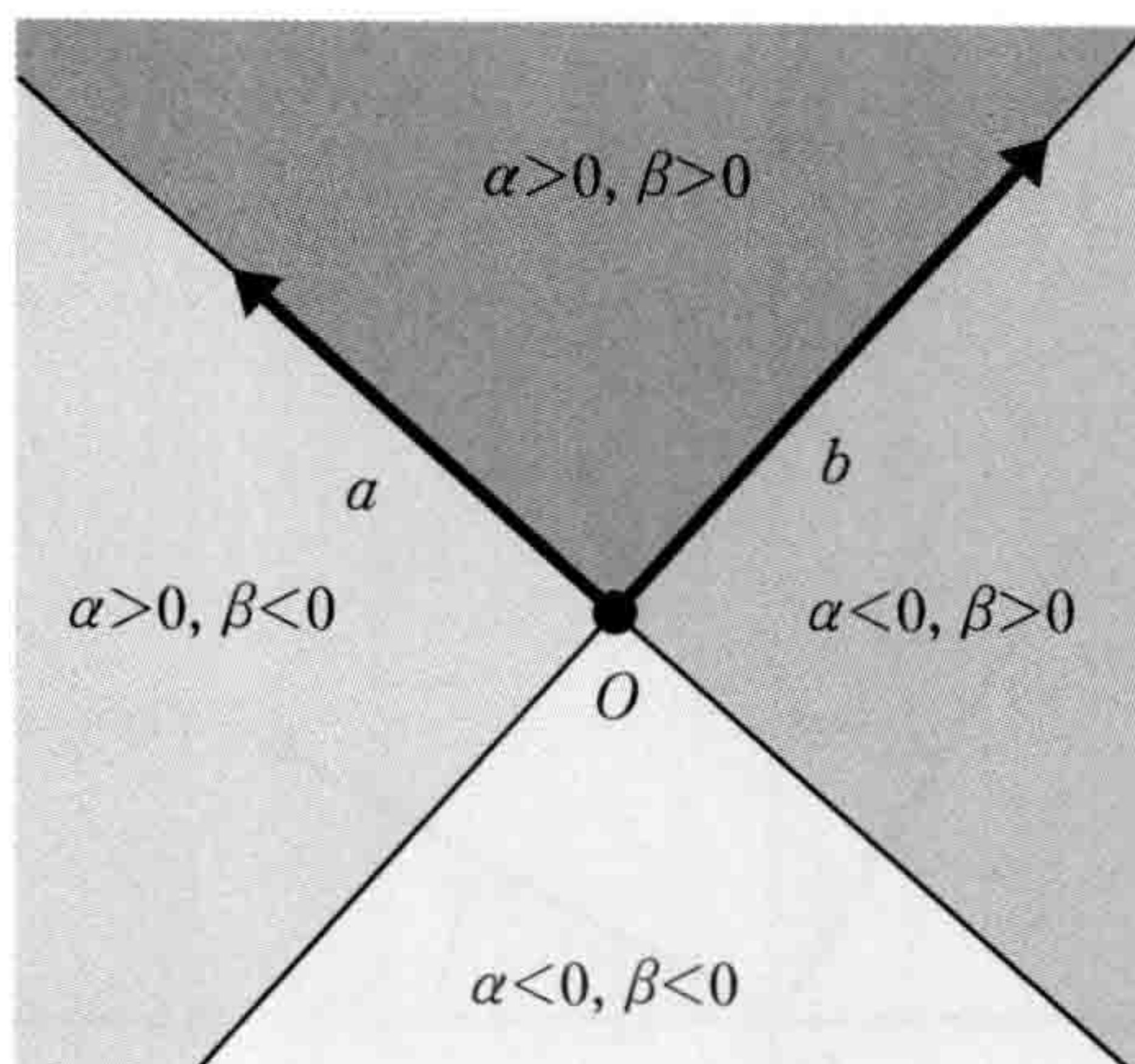
图6-5-4 二维向量中向量间位置关系的判定
