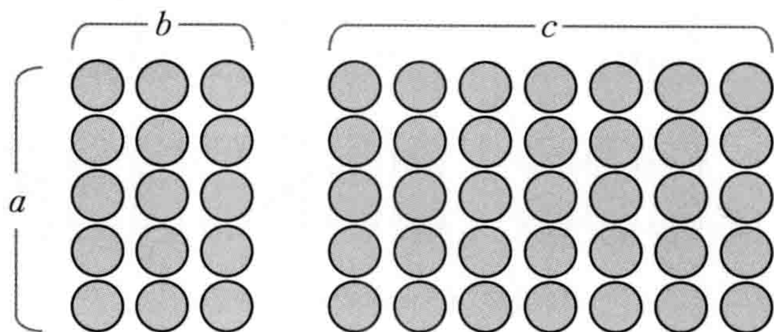
图6-2-1 5颗一袋的糖共3+7袋
