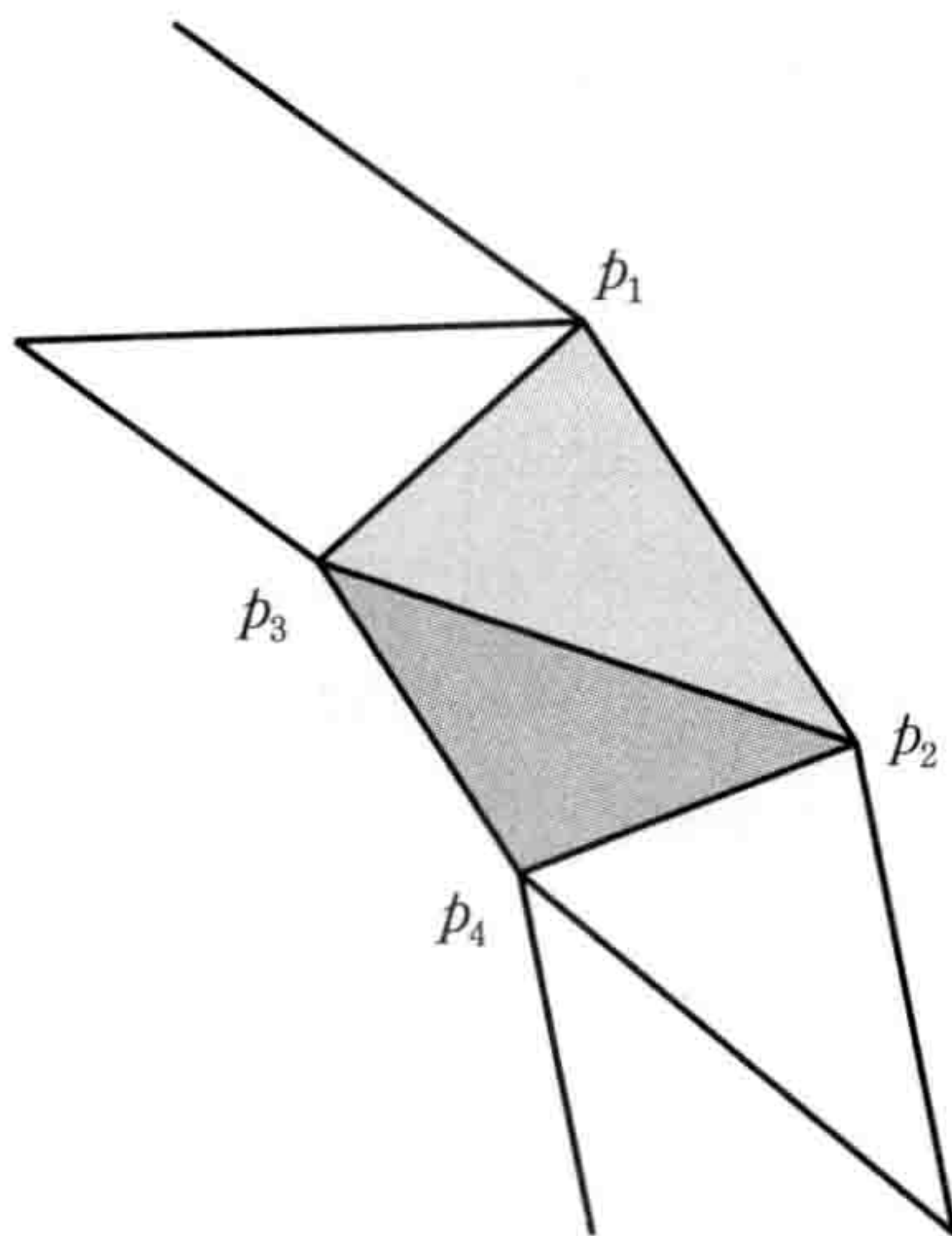
图4-3-3 将圆环分割后得到的图形为梯形
