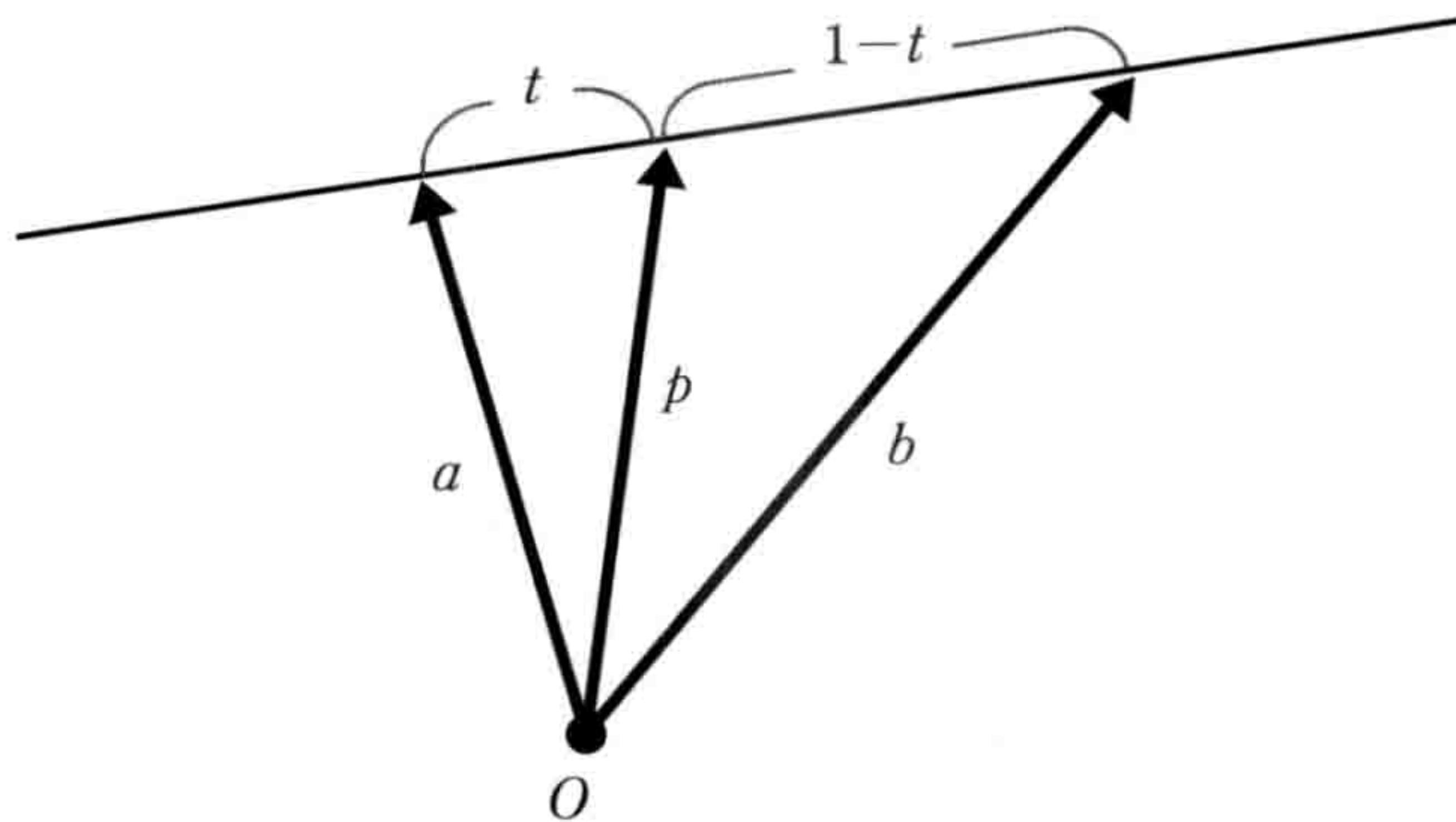
图6-5-3 向量的内分
