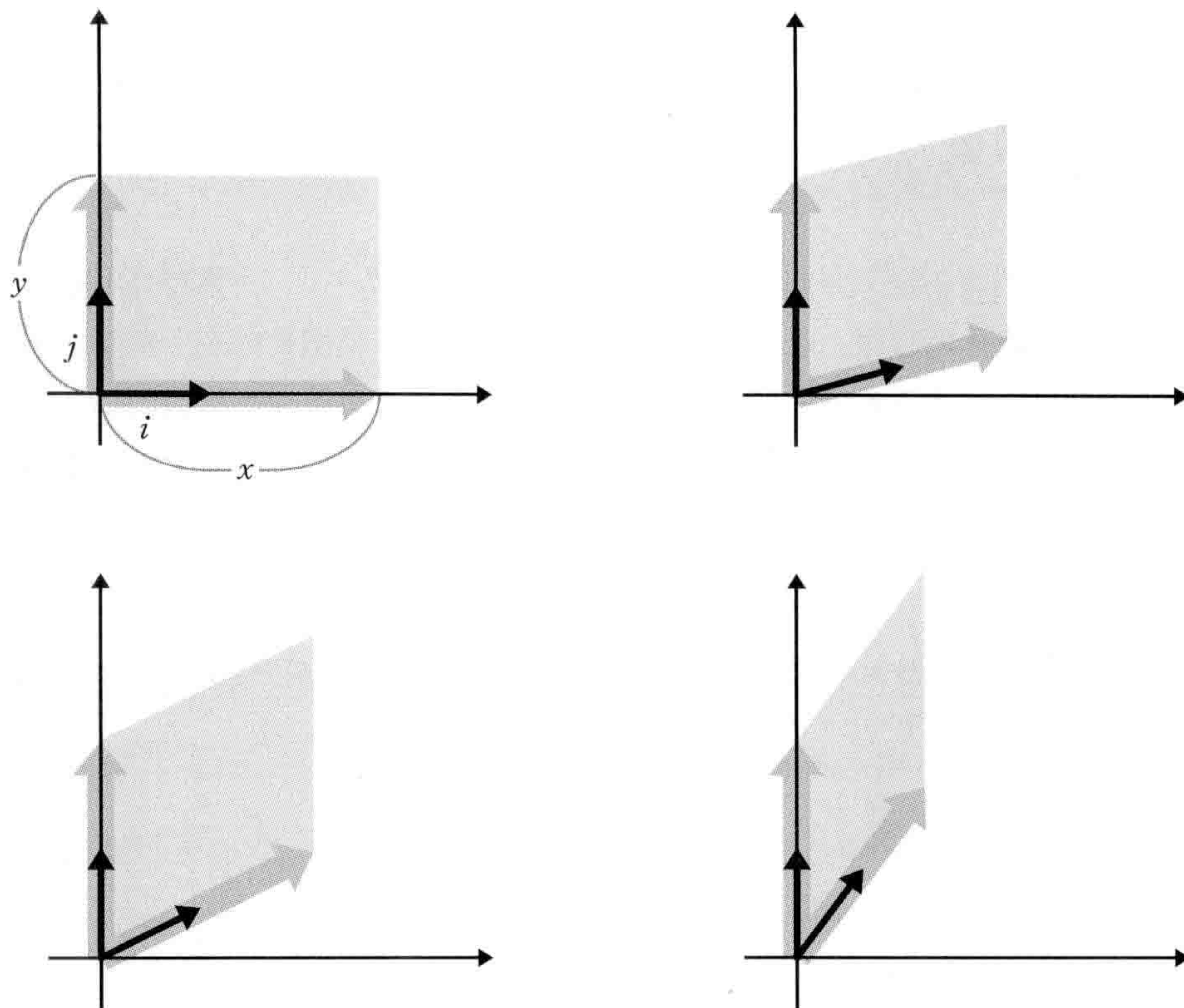
图4-1-3 切变
