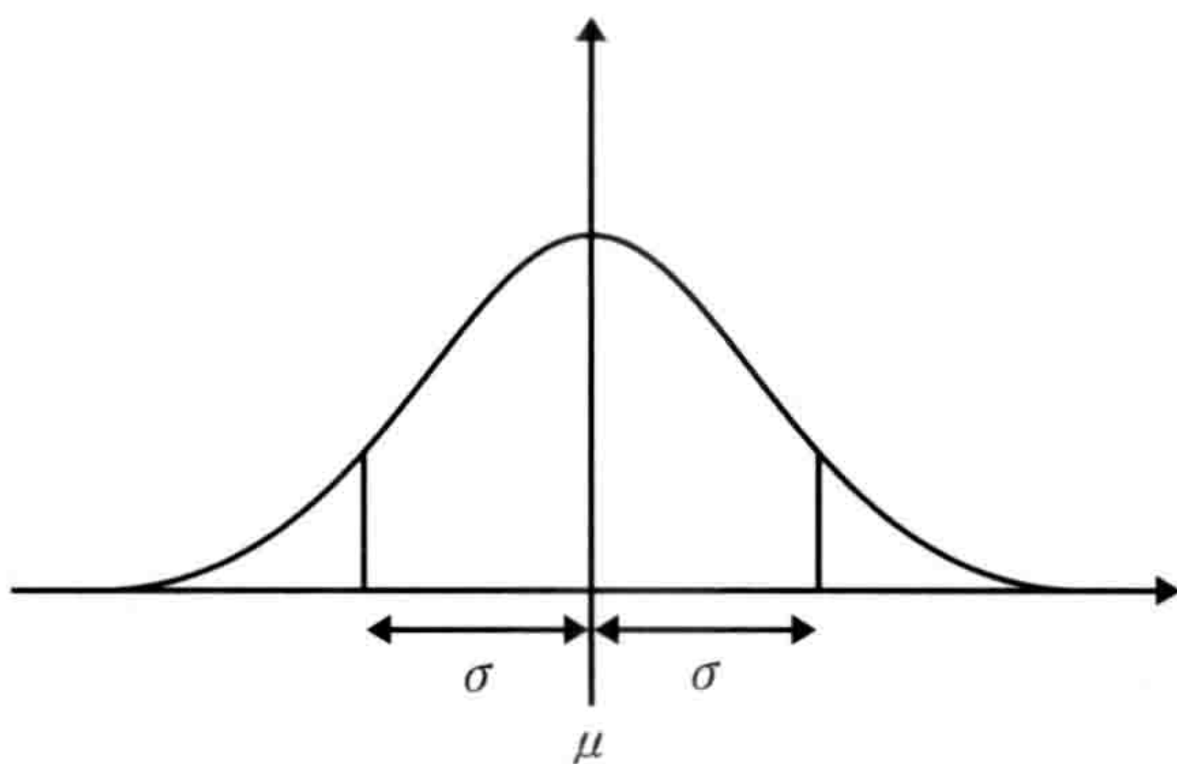
图1-5-2 正态分布的图像
