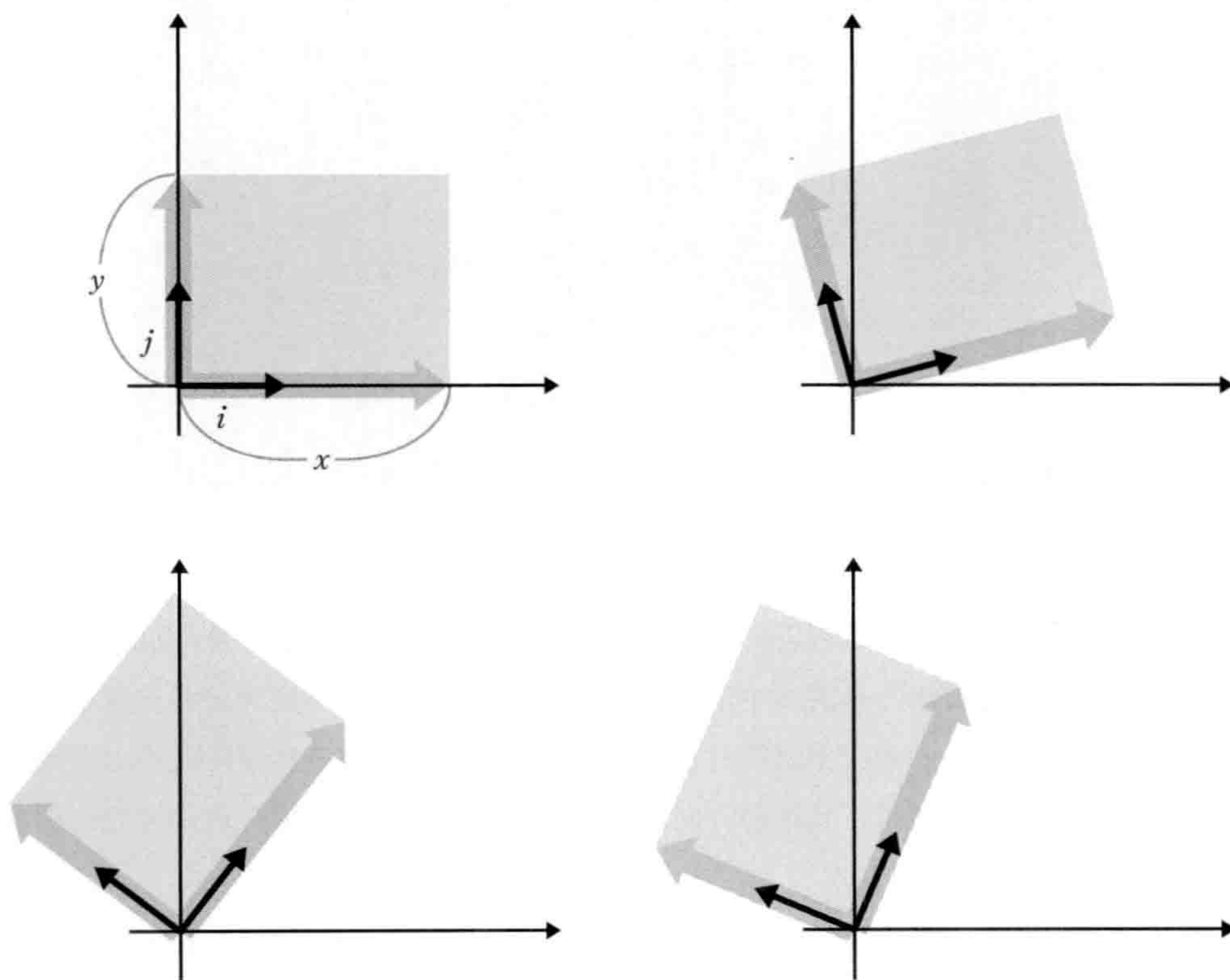
图4-1-2 通过 \mathbf{i} 与 \mathbf{j} 来实现物体的旋转
