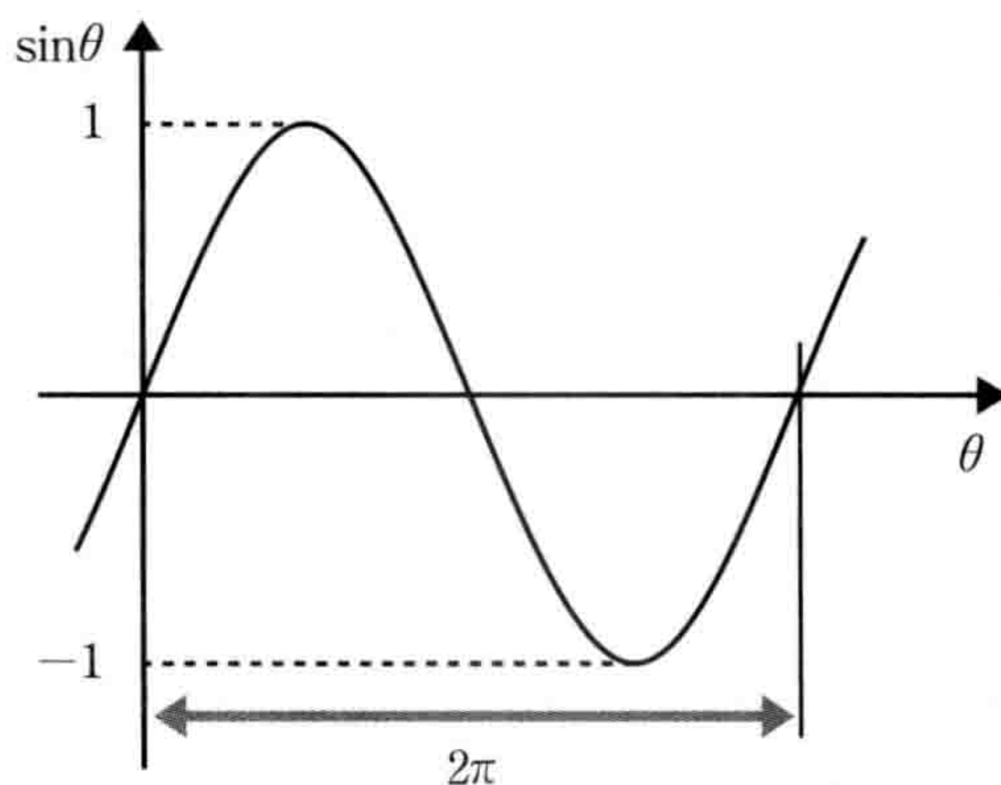
图2-4-4 正弦函数所绘制的图形
