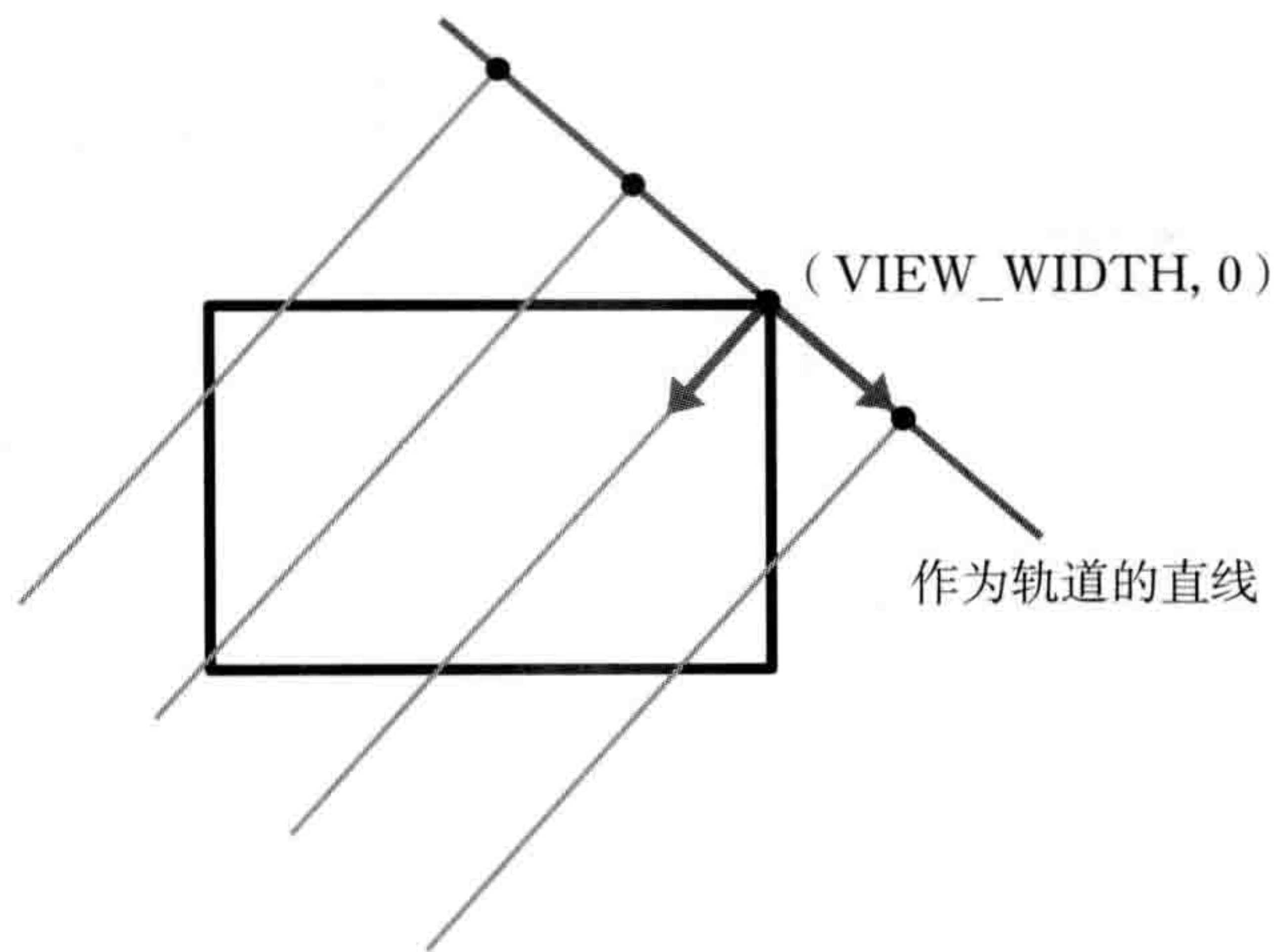
图5-2-2 以向量形式表示将画面沿45度角切分的直线
