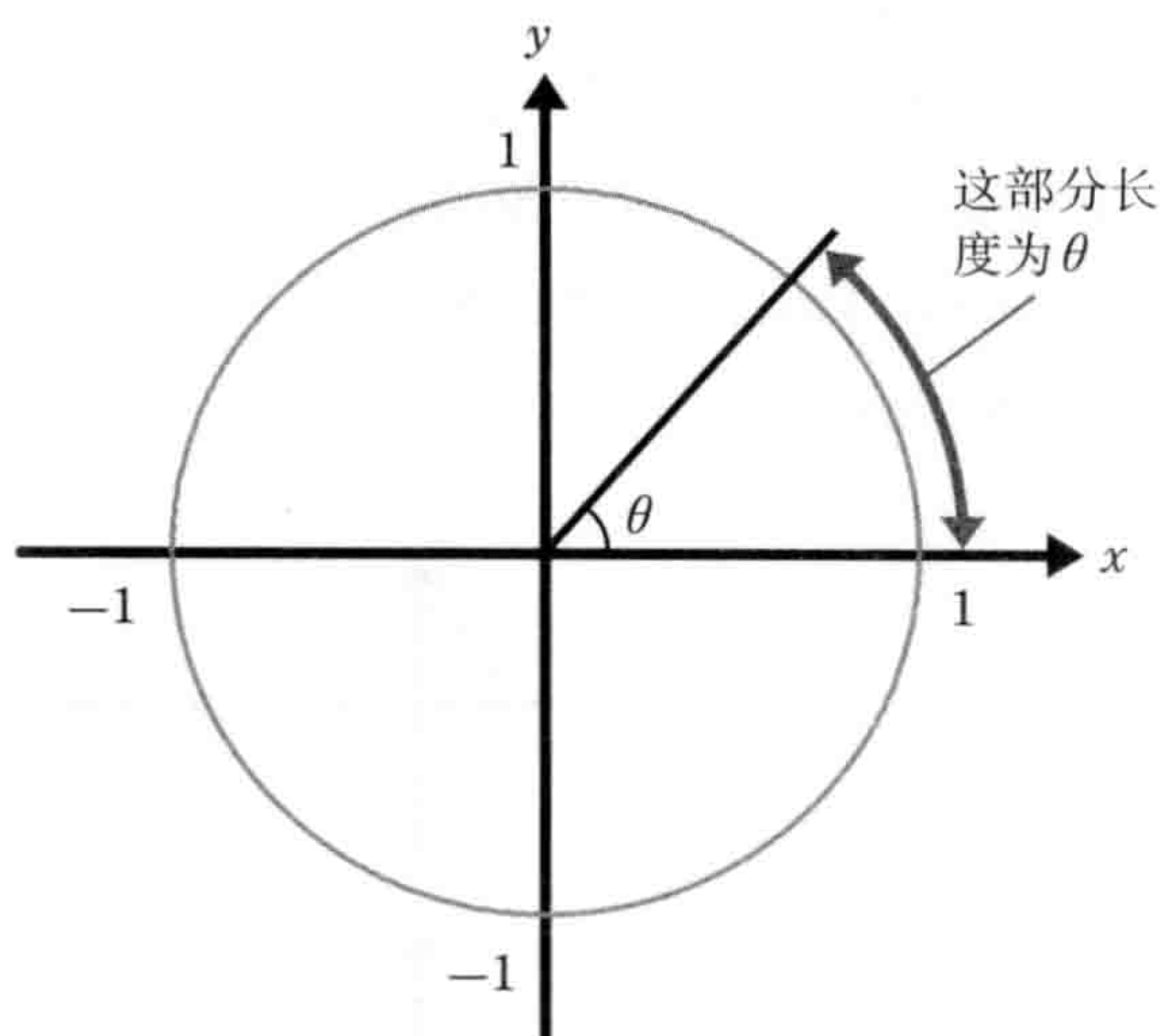
图6-4-5 弧度的定义
