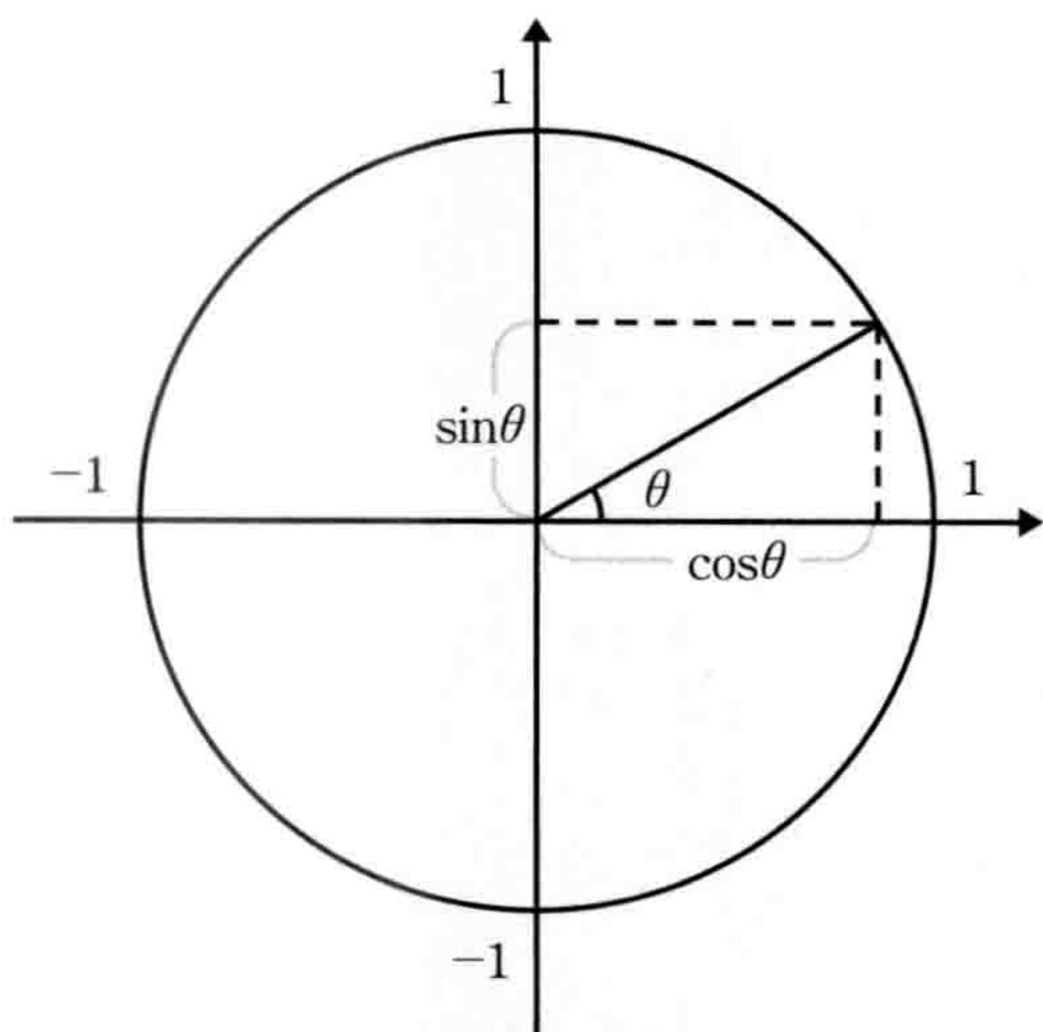
图 1-6-2 三角函数的定义
