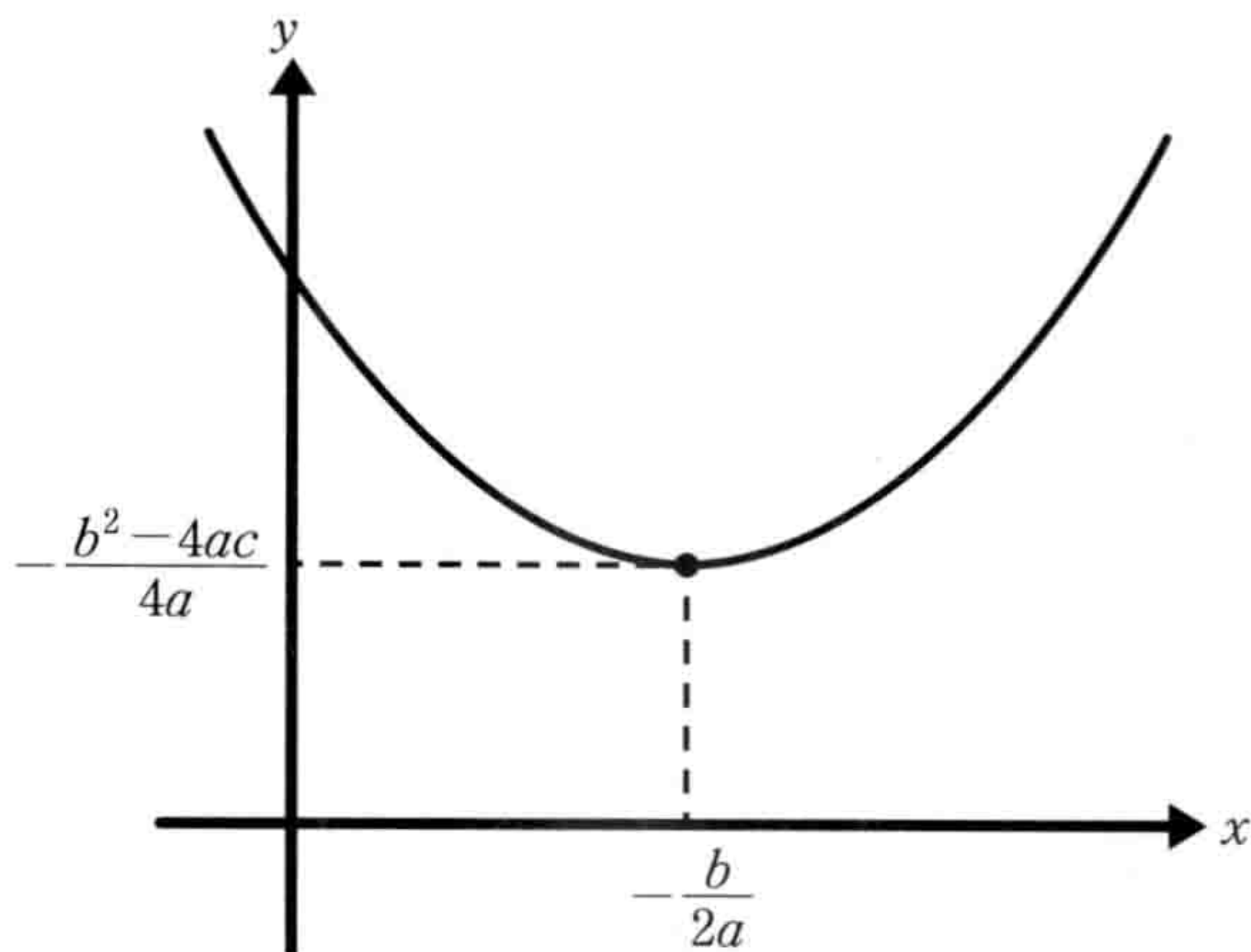
图6-3-2 平行移动的图形
