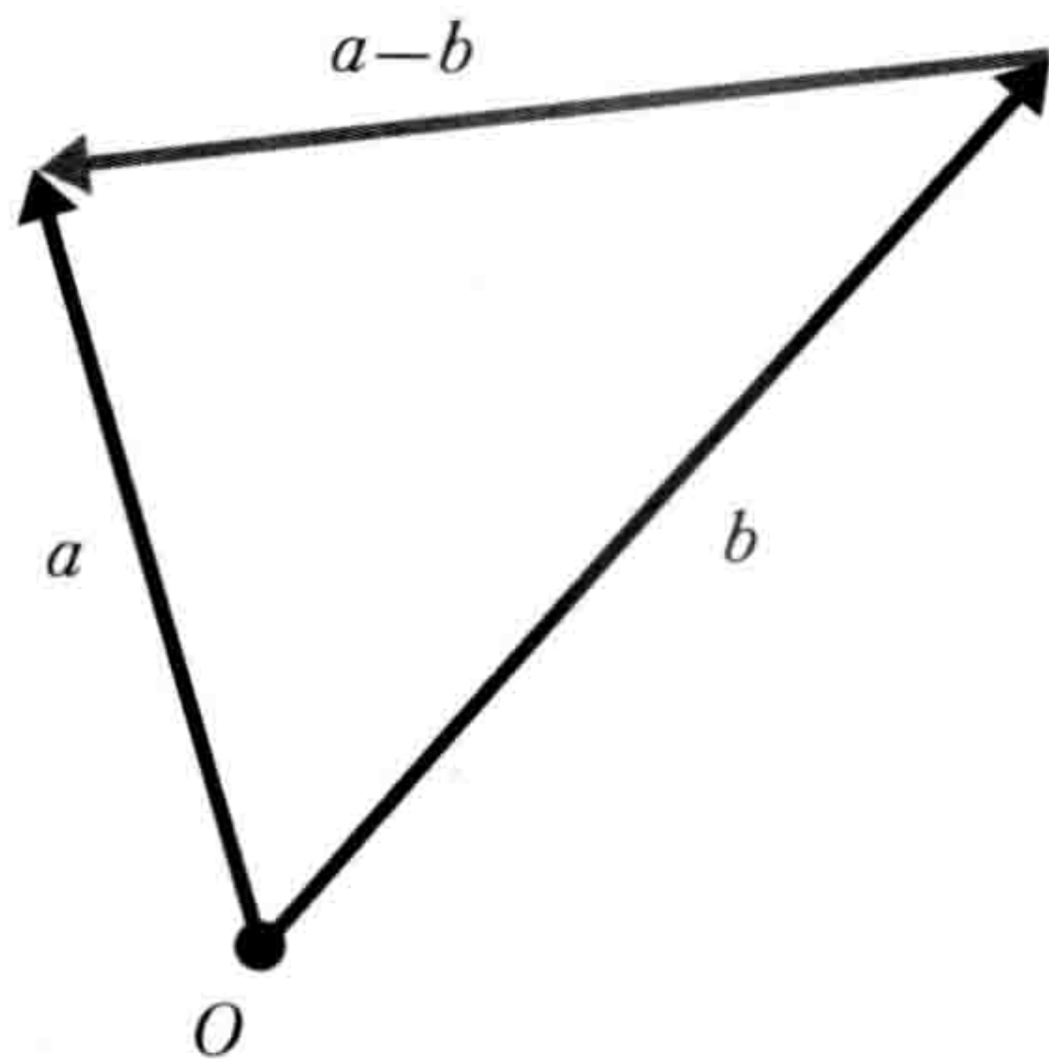
图 6-5-2 向量的减法运算
