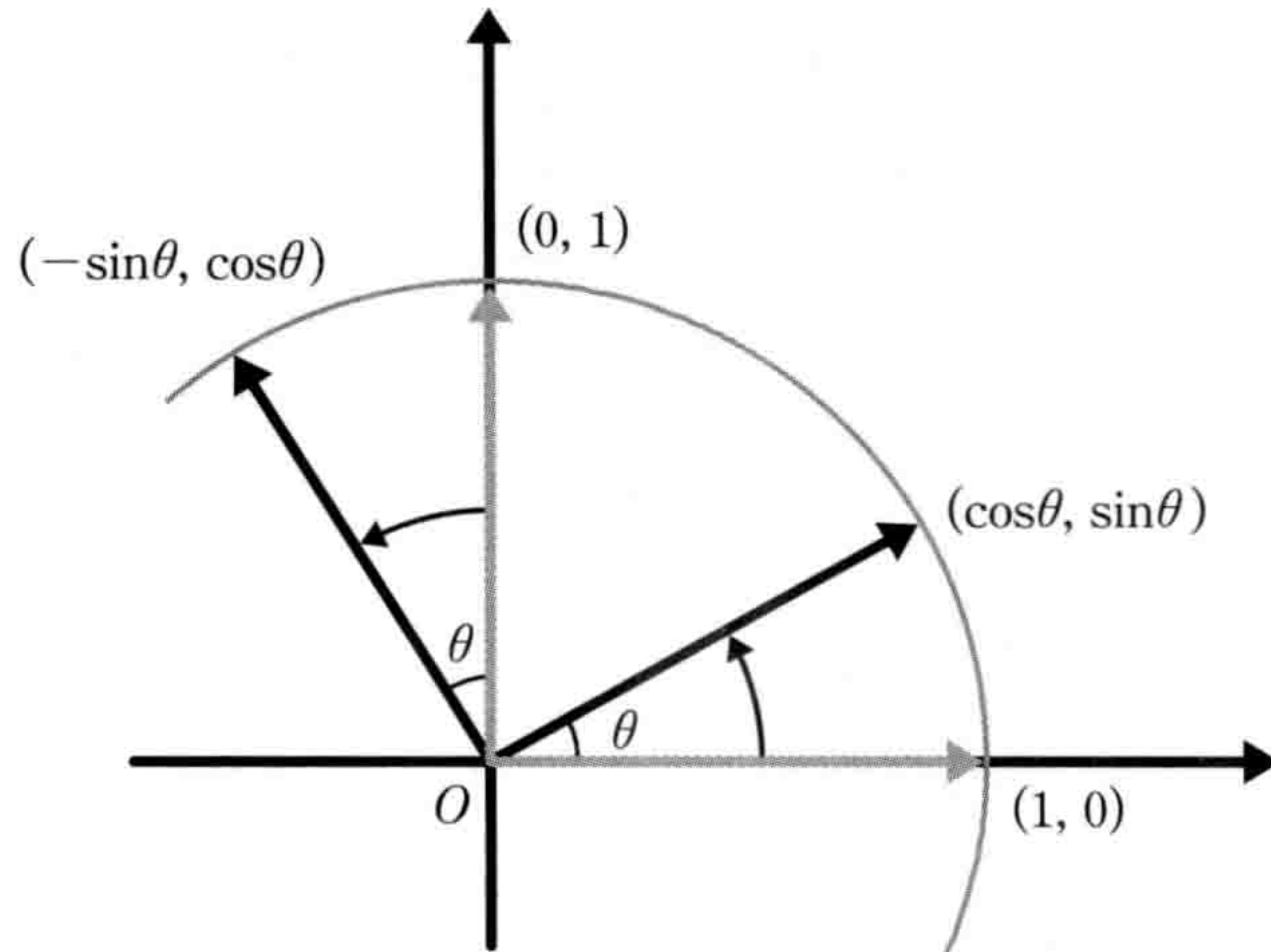
图6-5-5 向量的旋转
