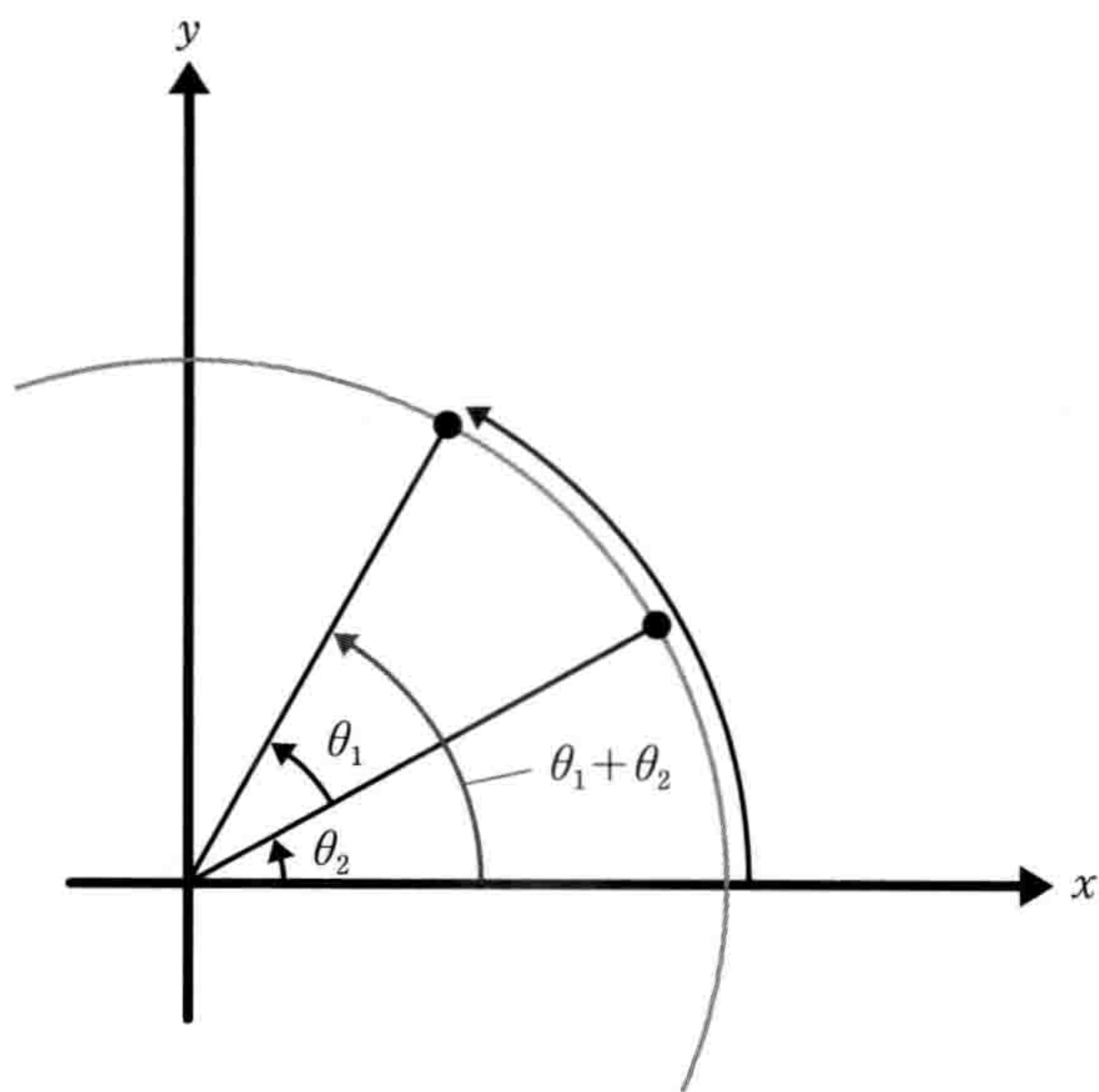
图6-4-8 表示加法定理的图
