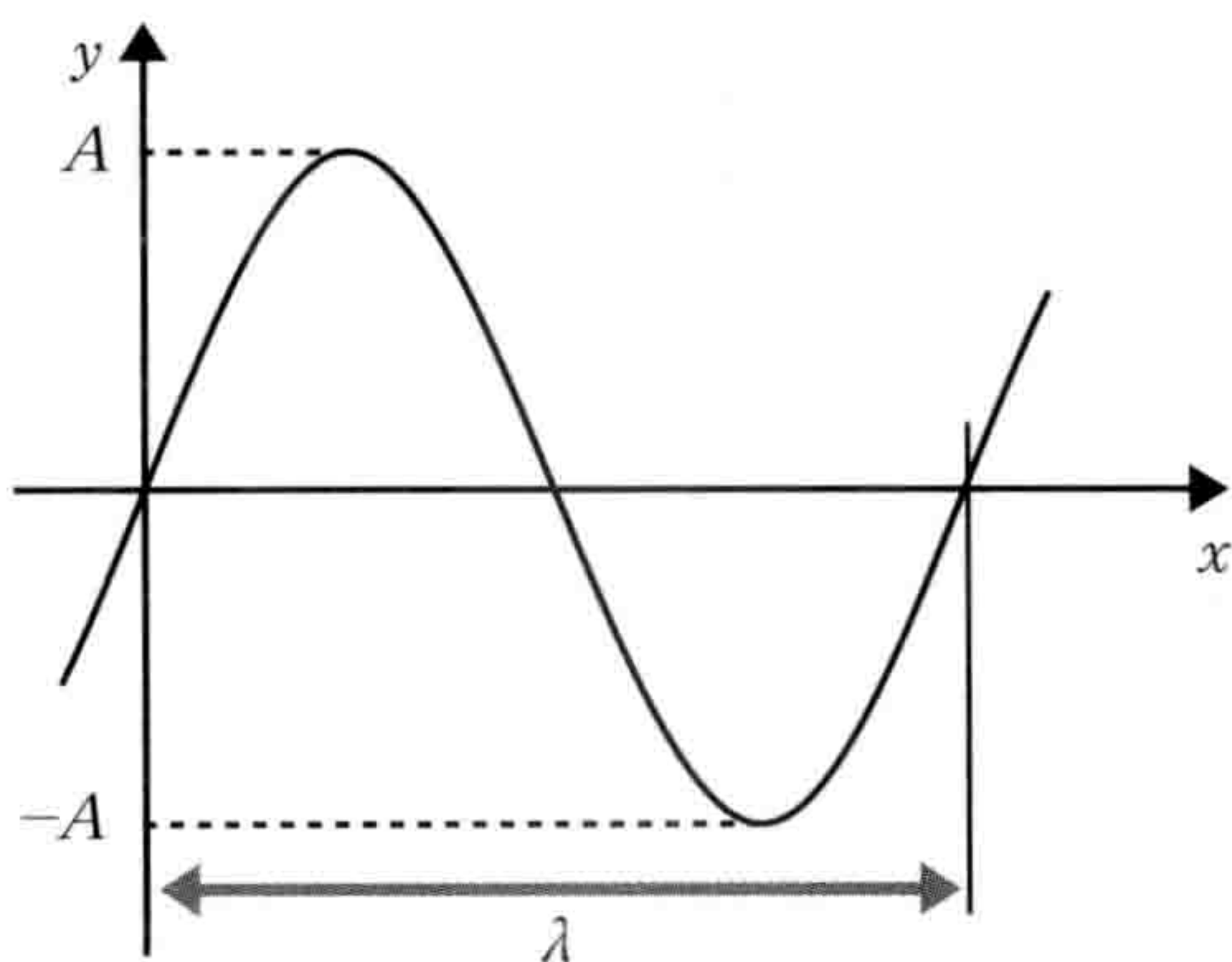
图2-4-5 正弦波的振幅 A 与波长 \lambda
