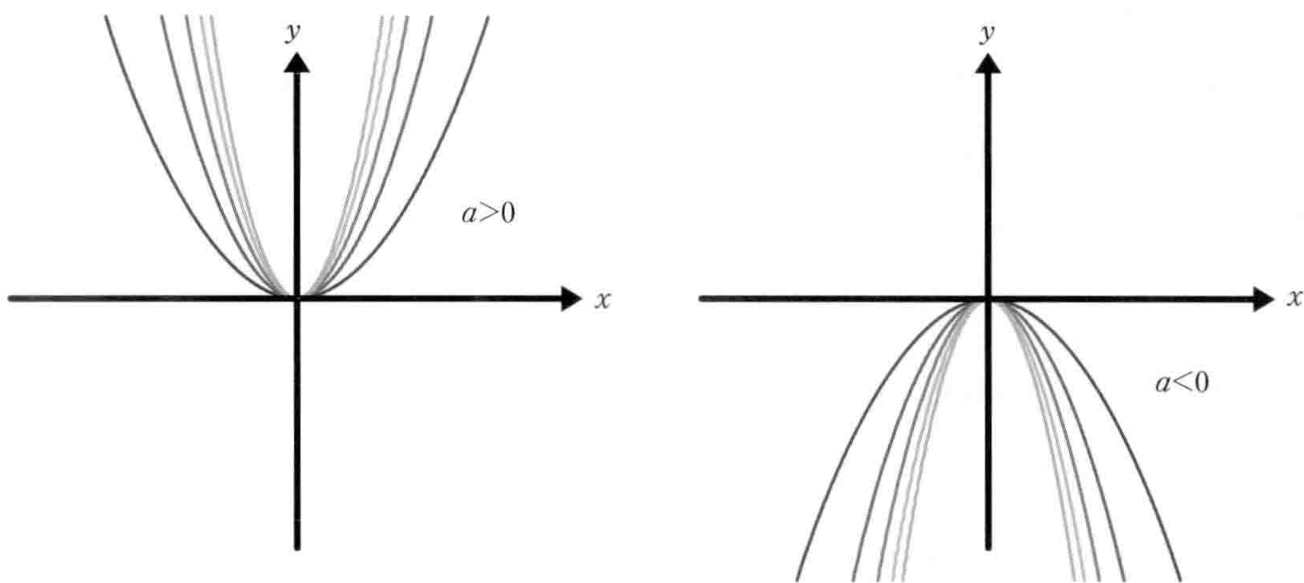
图6-3-1 最简单的二次函数的图形(抛物线)
