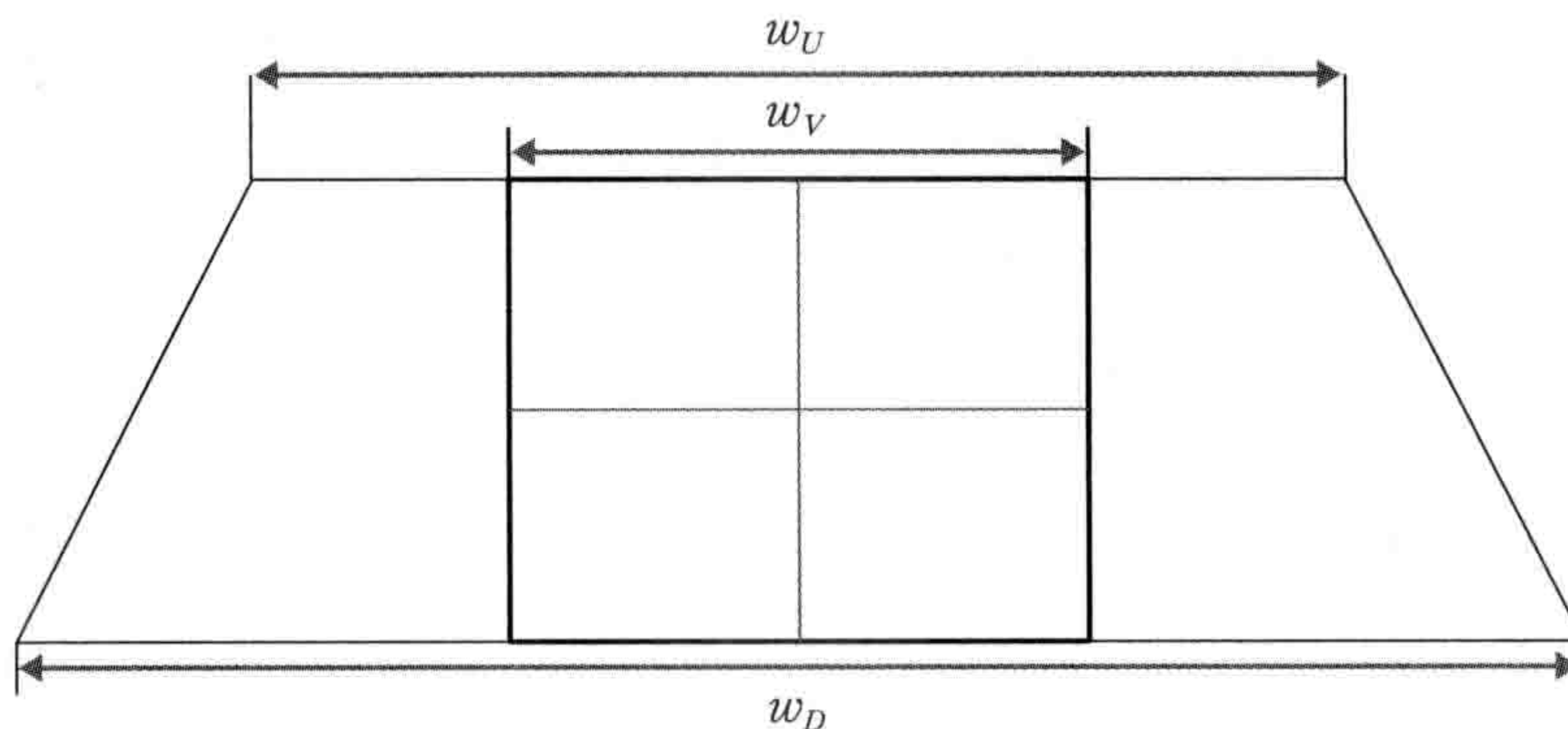
图 2-5-2 等式各要素与图形的对应关系
