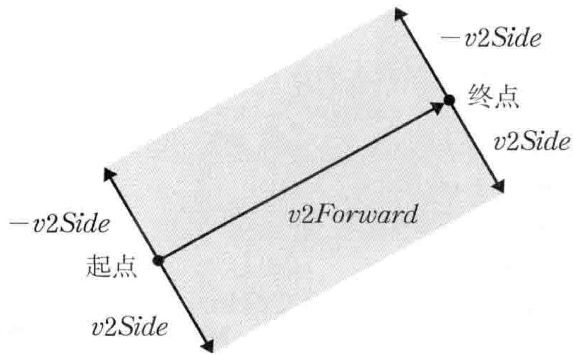
图4-2-2 通过起点、终点及向量计算图形的四个角
